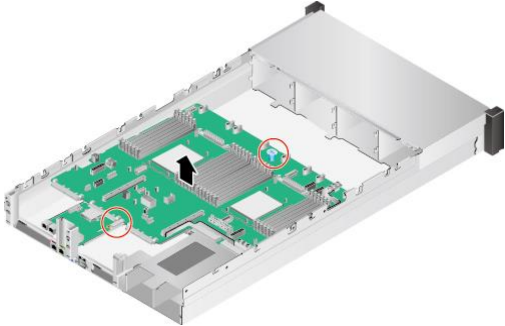
图6-99 拆卸主板
