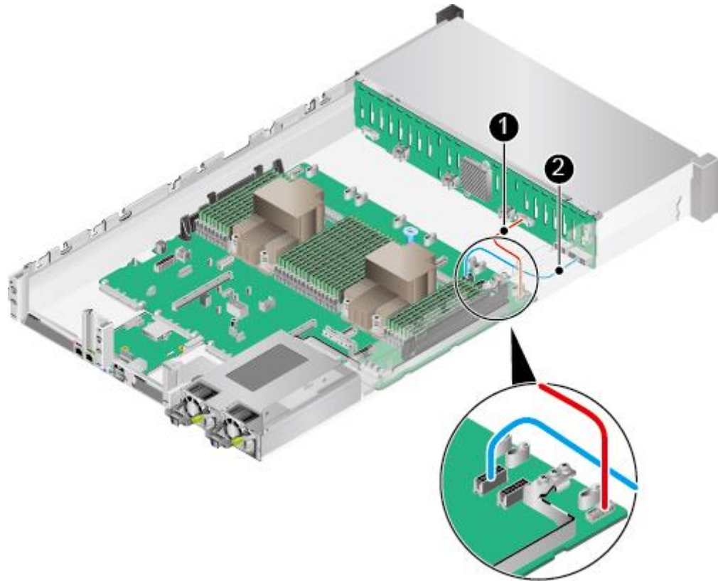
图4-10 前置硬盘背板的电源线和点灯信号线
