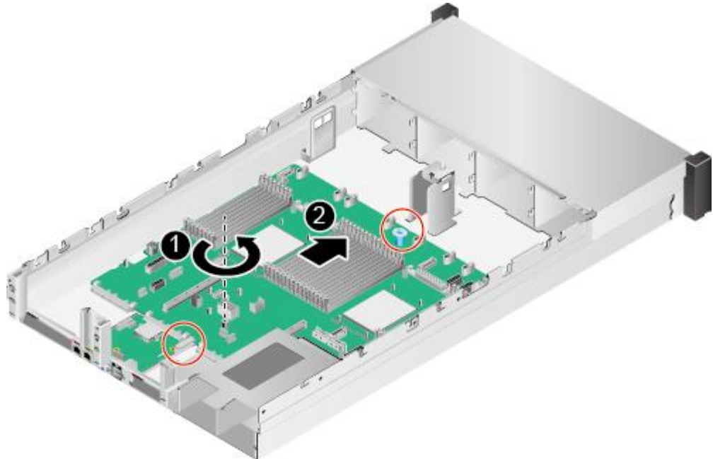
图6-98 拆卸主板
