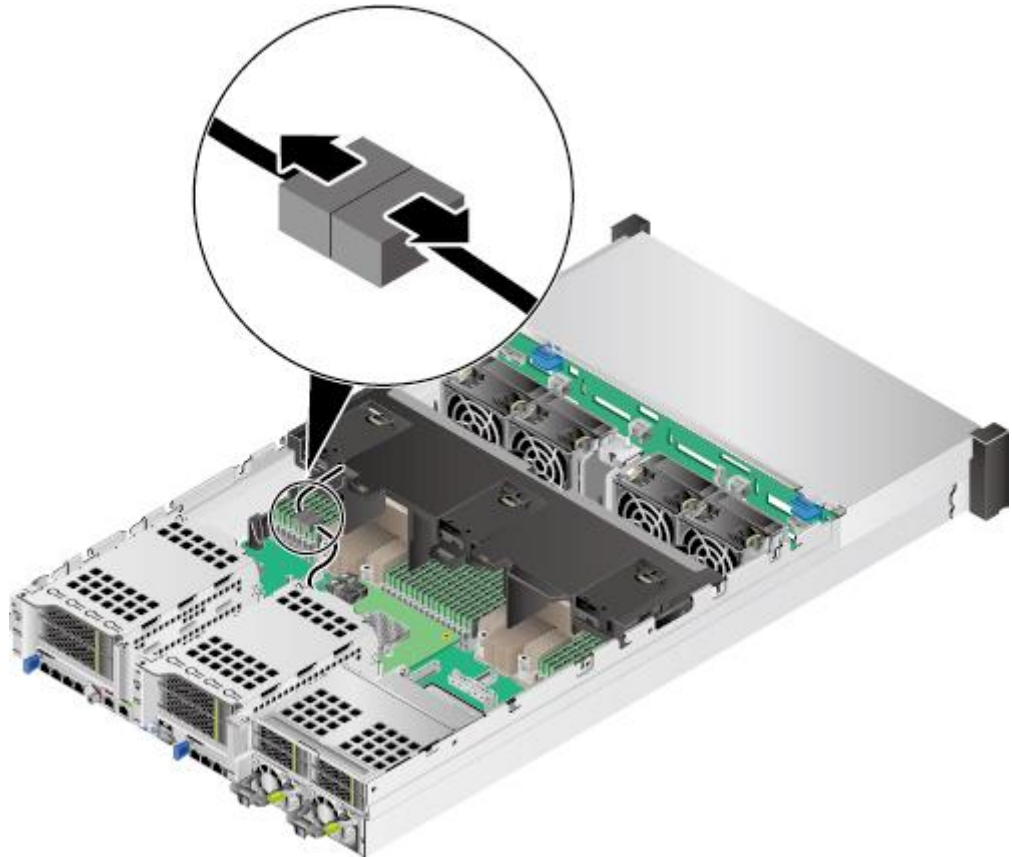
图6-35 拆卸超级电容线缆
