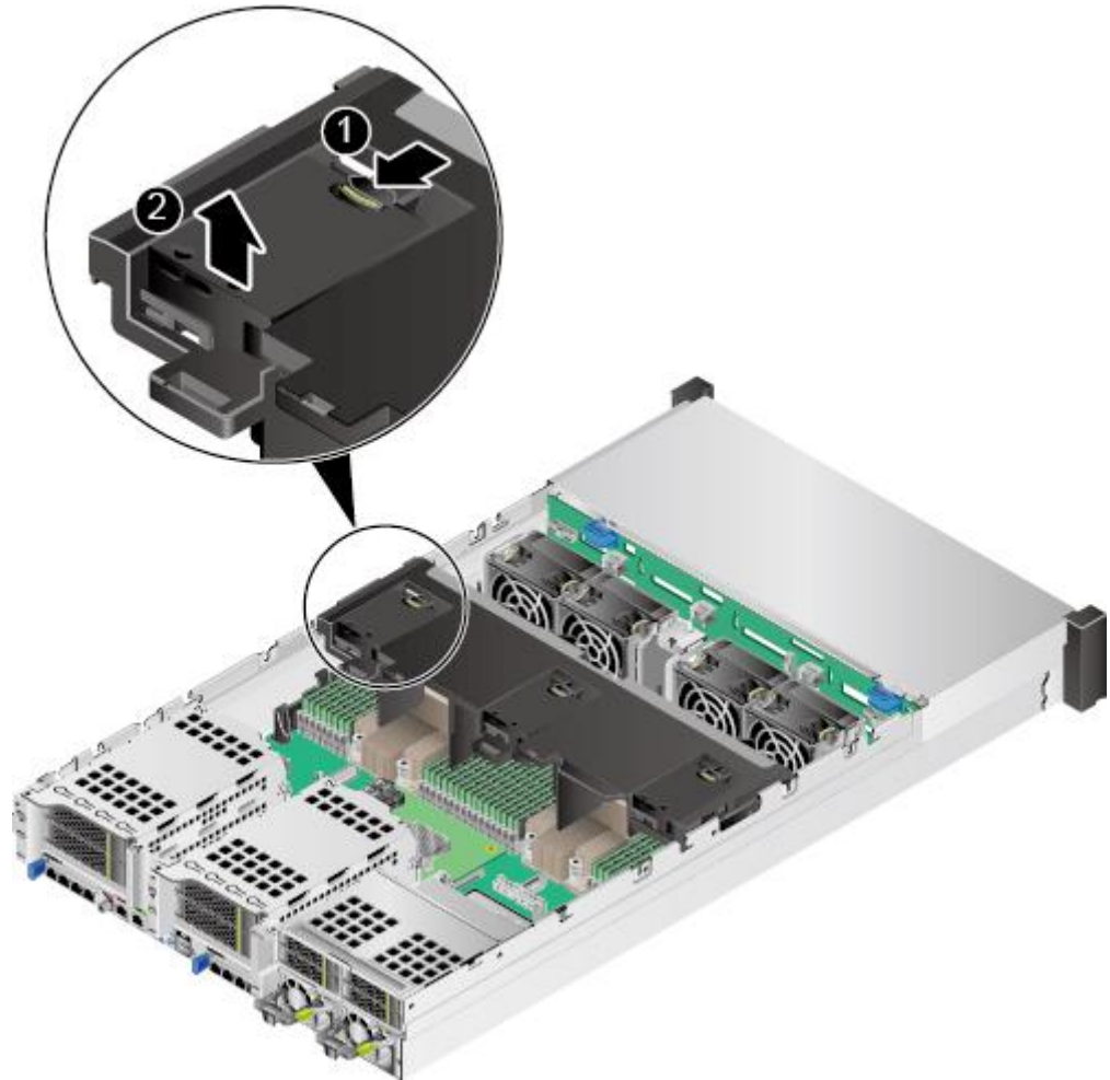
图6-66 拆卸超级电容支架
