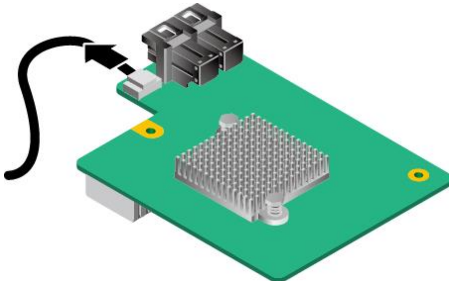
图6-65 拔出超级电容线缆
