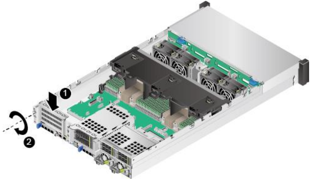
图6-45 安装空闲挡板（1）
