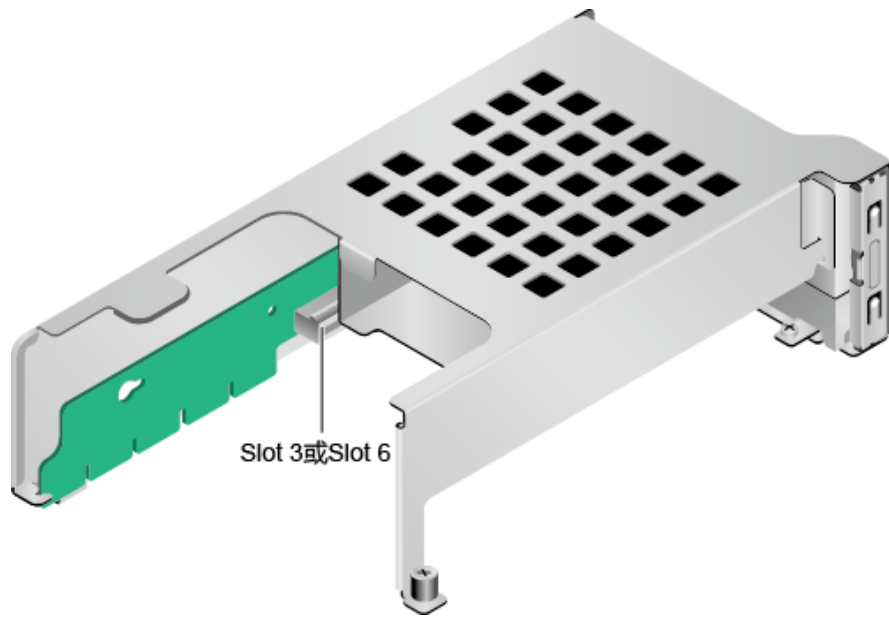
图3-32 Riser 卡 4 (1x16)
