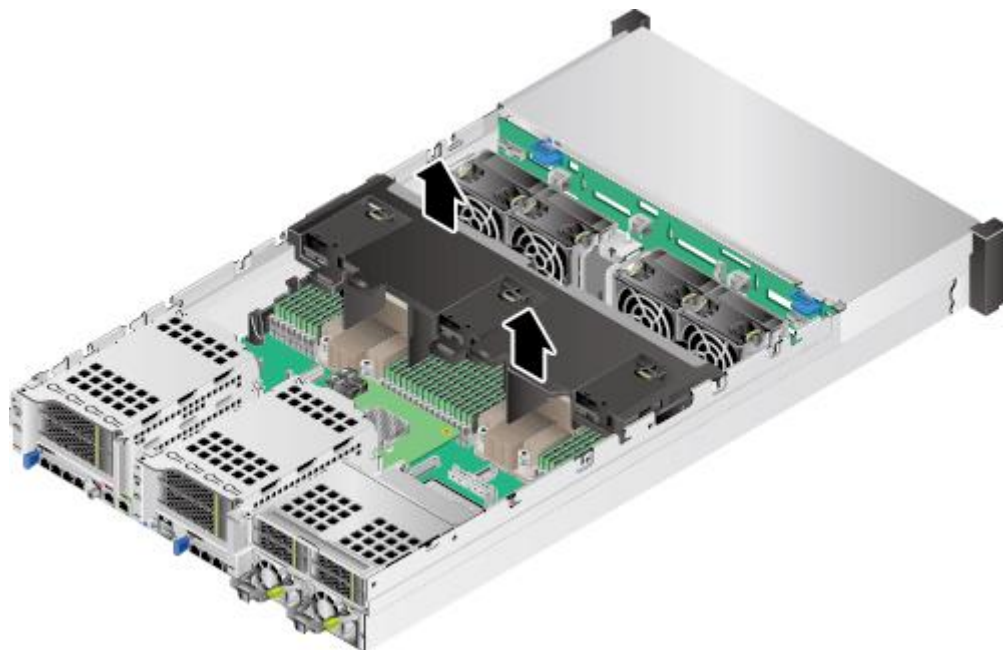
图6-36 拆卸导风罩
