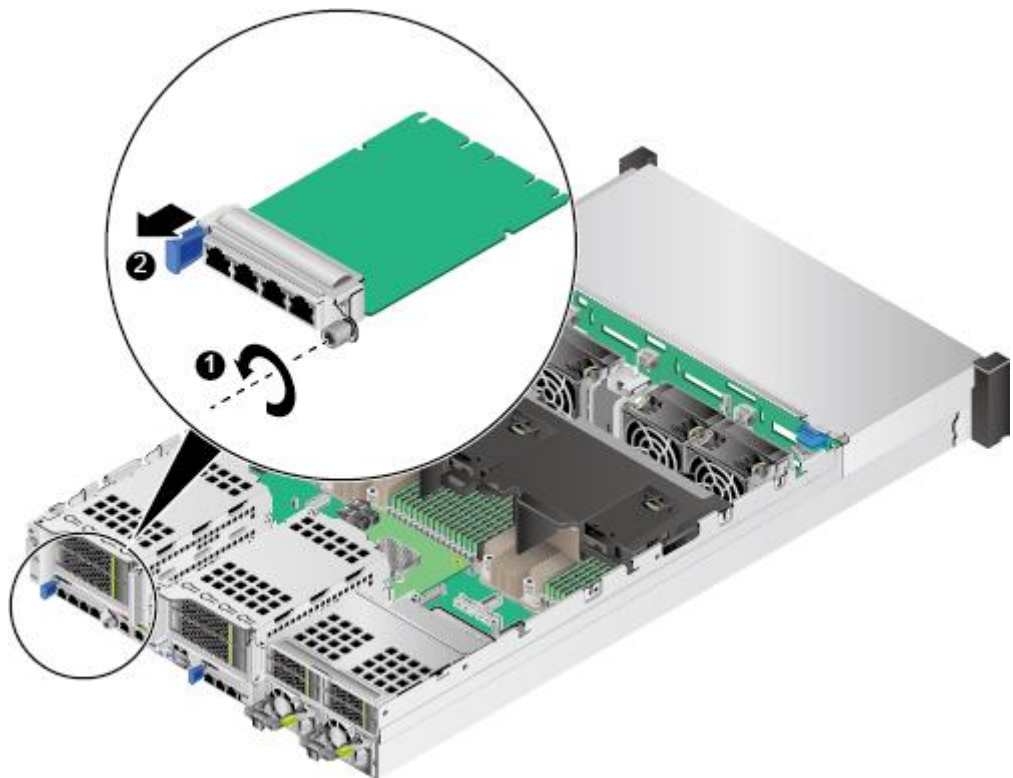
图6-74 拆卸灵活 IO 卡
