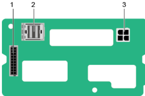
图3-24 2x3.5 英寸后置硬盘背板
