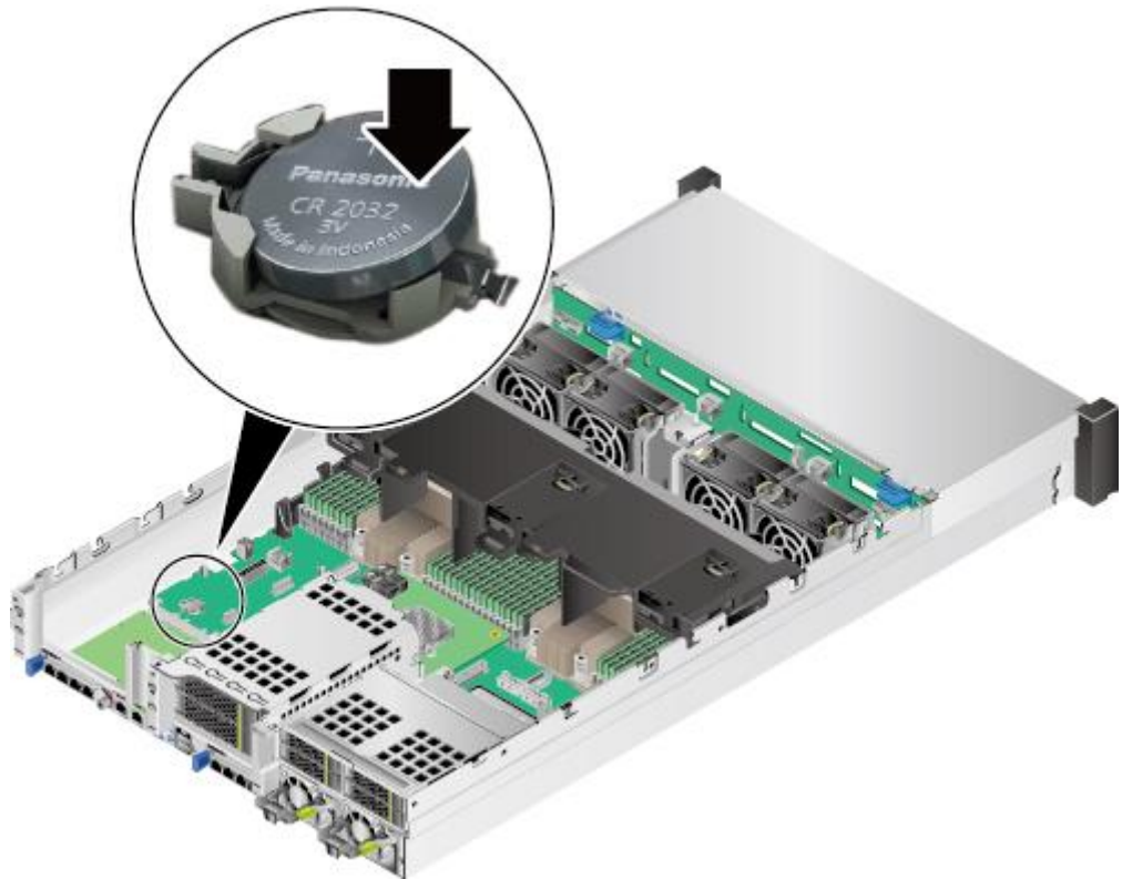
图6-60 安装电池
