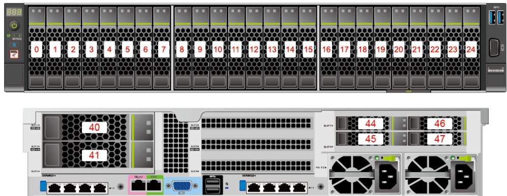
图3-14 25x2.5 英寸硬盘 EXP 配置硬盘编号
