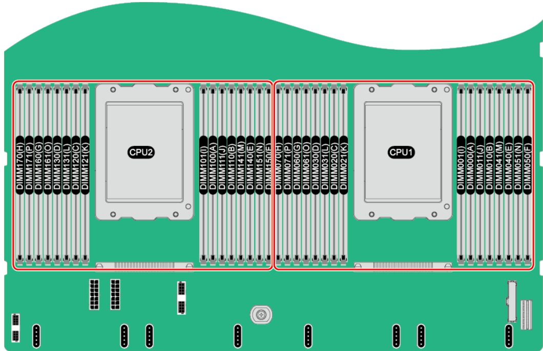
图3-28 内存槽位编号
