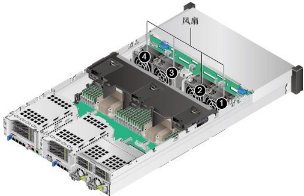
图3-37 风扇位置图
