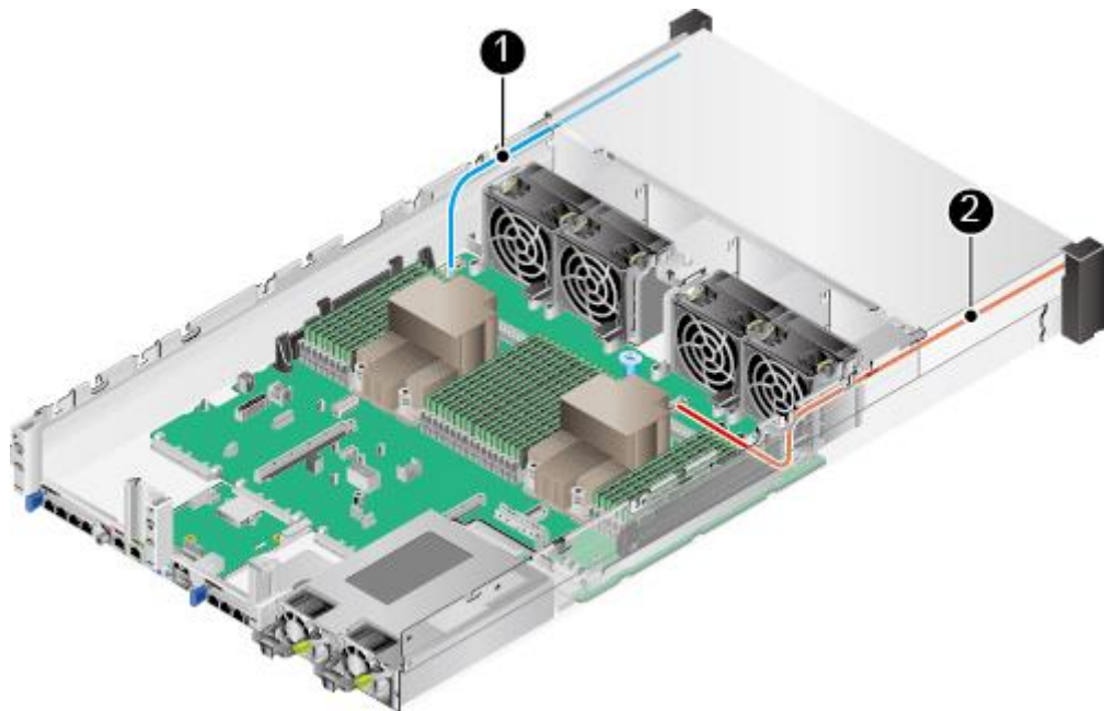
图4-9 左右挂耳连线
