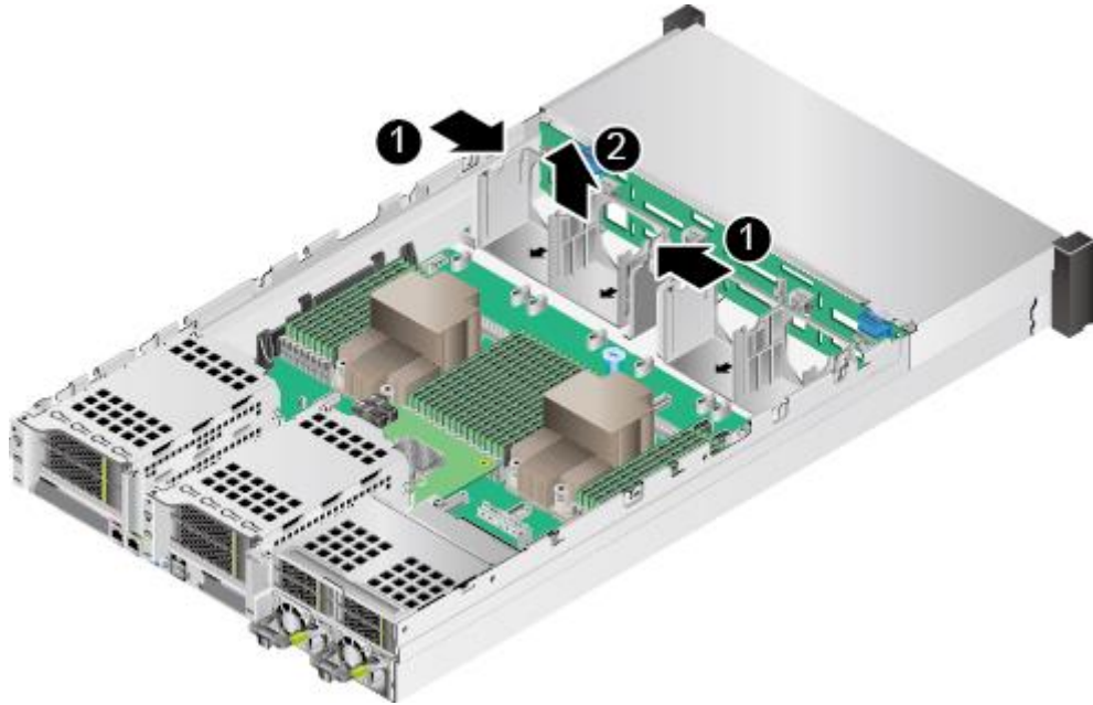
图6-94 拆卸风扇支架
