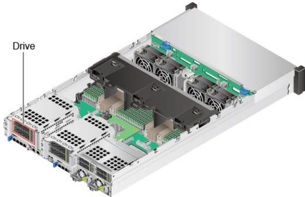
图6-82 硬盘位置
