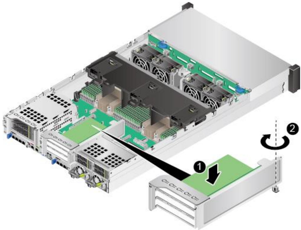
图6-52 安装 Riser 模组 2
