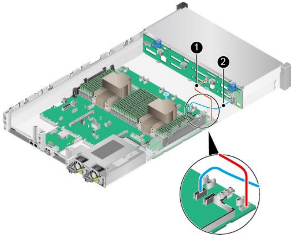
图4-6 前置硬盘背板的电源线和点灯信号线
