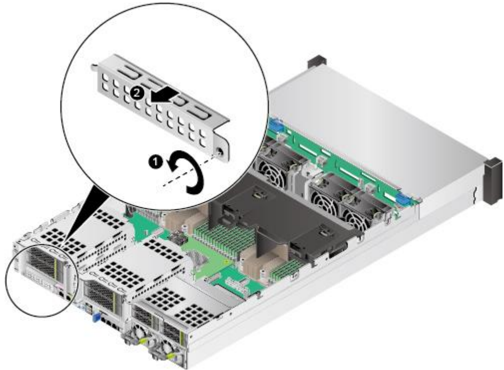
图6-76 拆卸灵活 IO 卡空闲挡板
