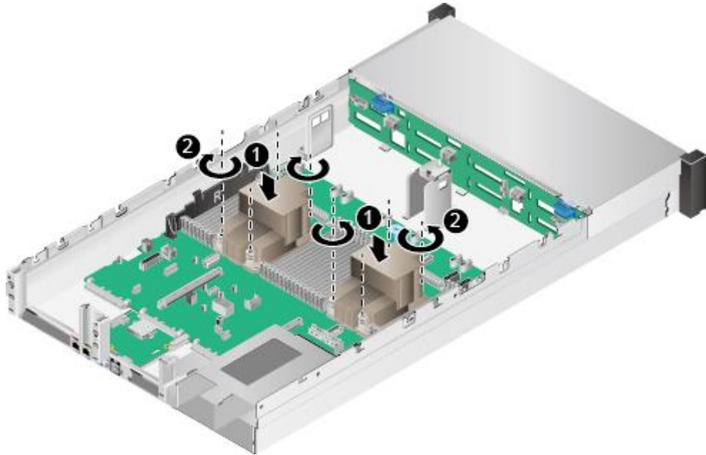
图6-106 安装 CPU 散热器
