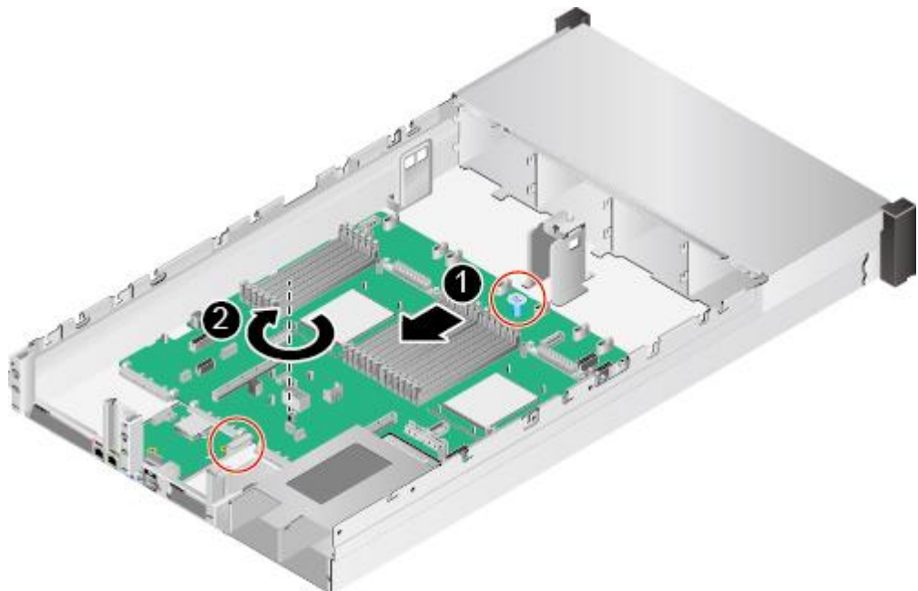
图6-101 安装主板
