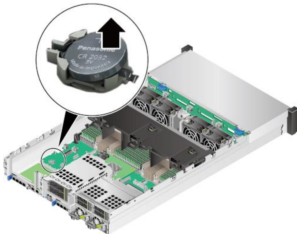
图6-59 拆卸电池
