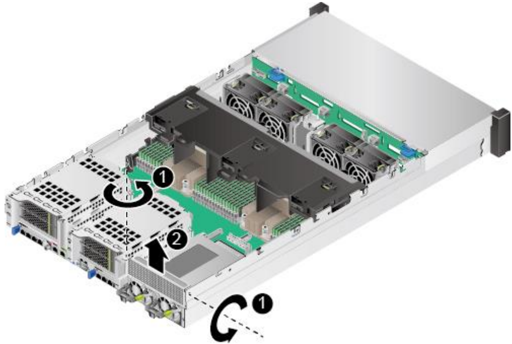
图6-50 拆卸空闲挡板（3）
