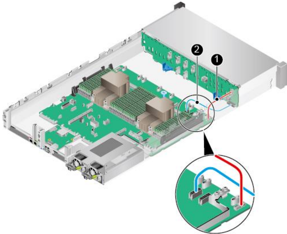
图4-14 前置硬盘背板的电源线和点灯信号线
