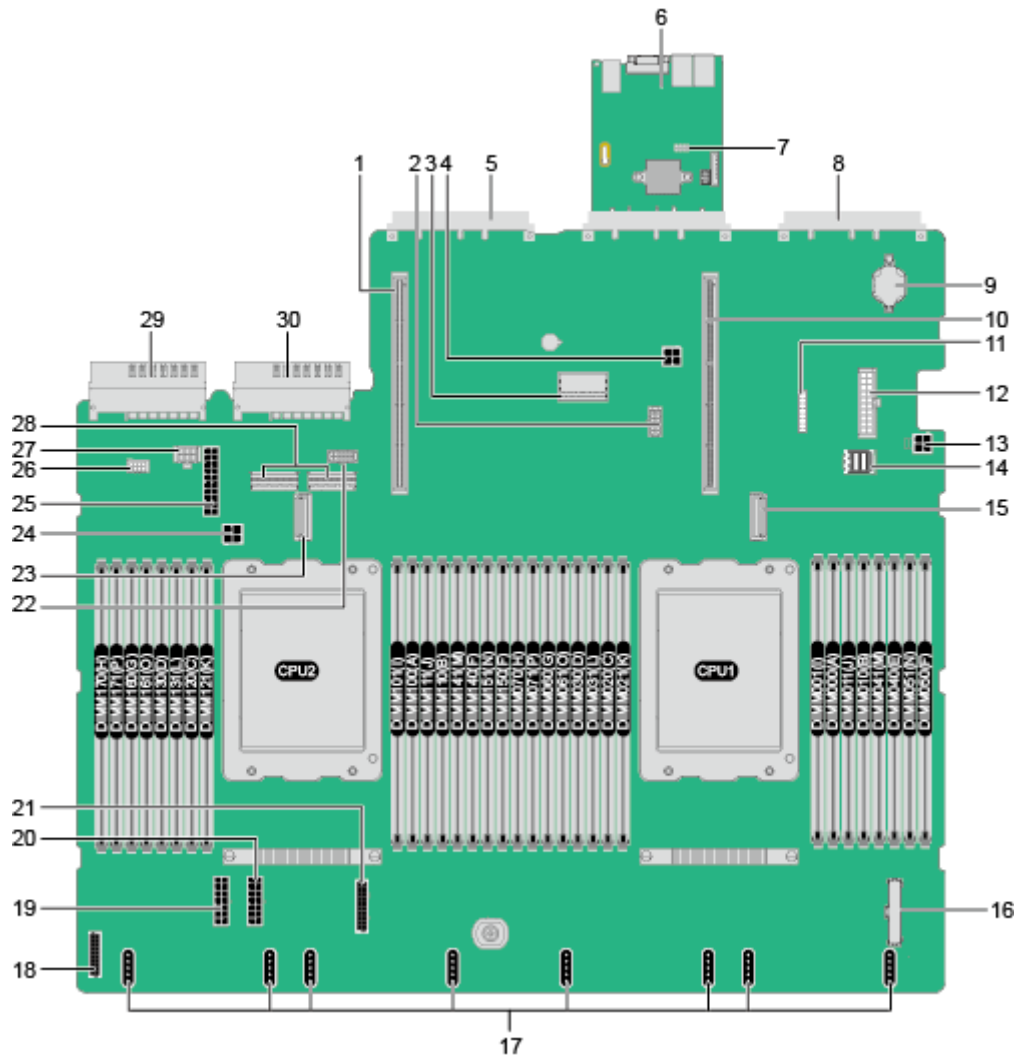
图3-27 主板和 iBMC 插卡接口
