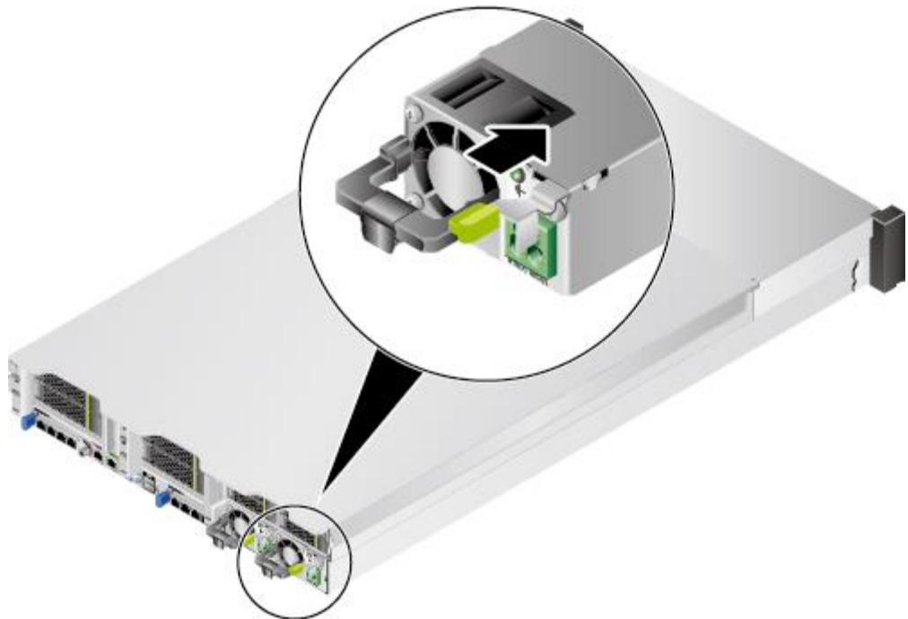
图6-31 安装电源模块
