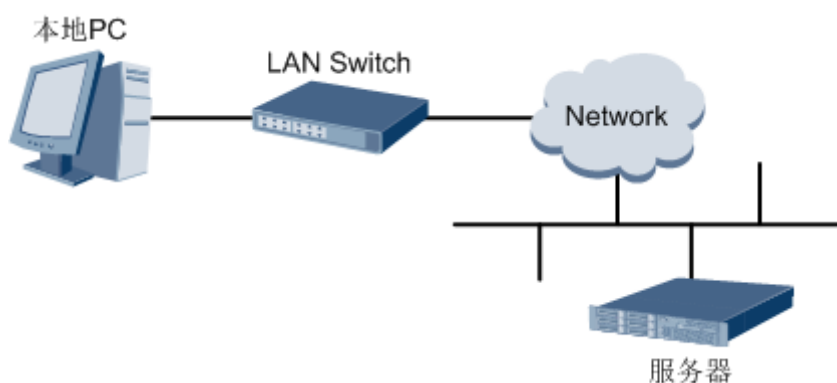
图8-4 组网图
