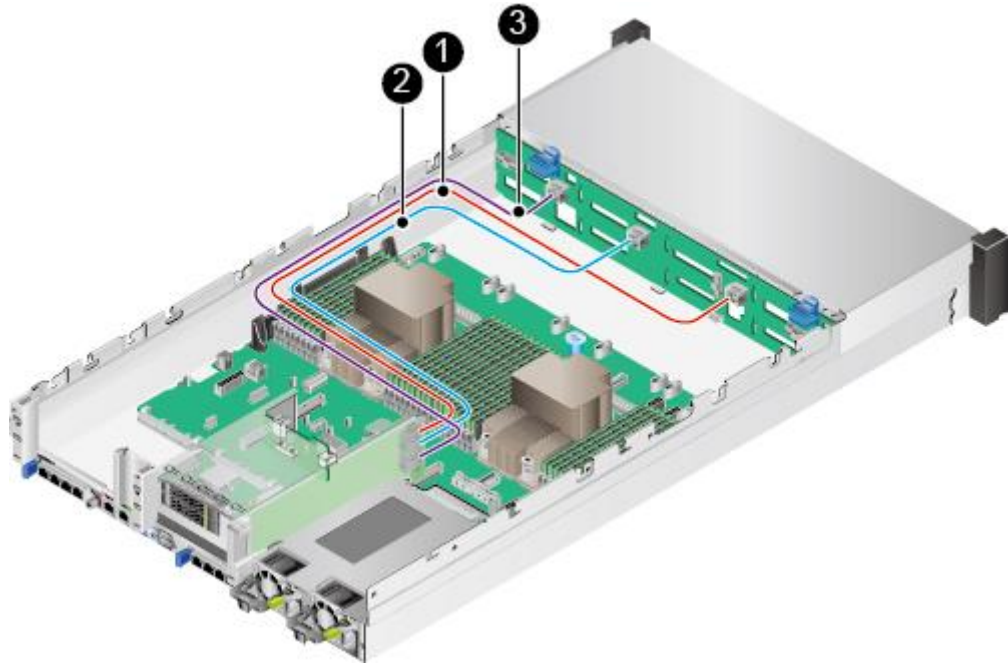
图4-7 前置硬盘背板的 SAS 信号线
