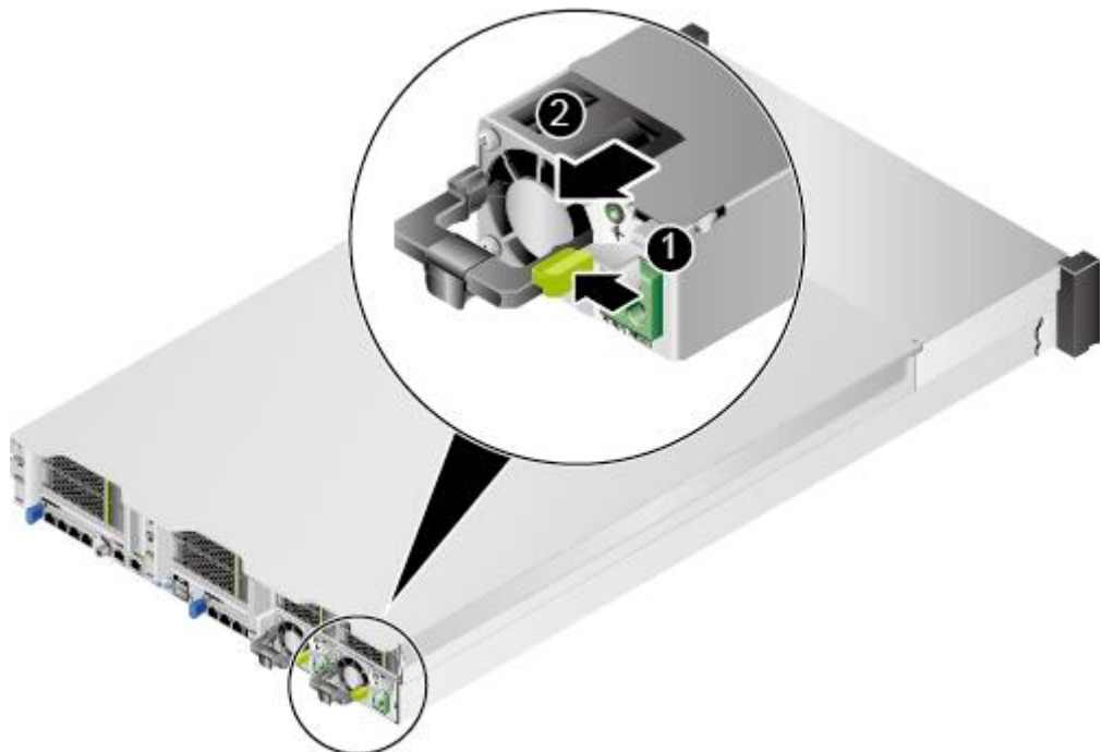
图6-28 拆卸电源模块
