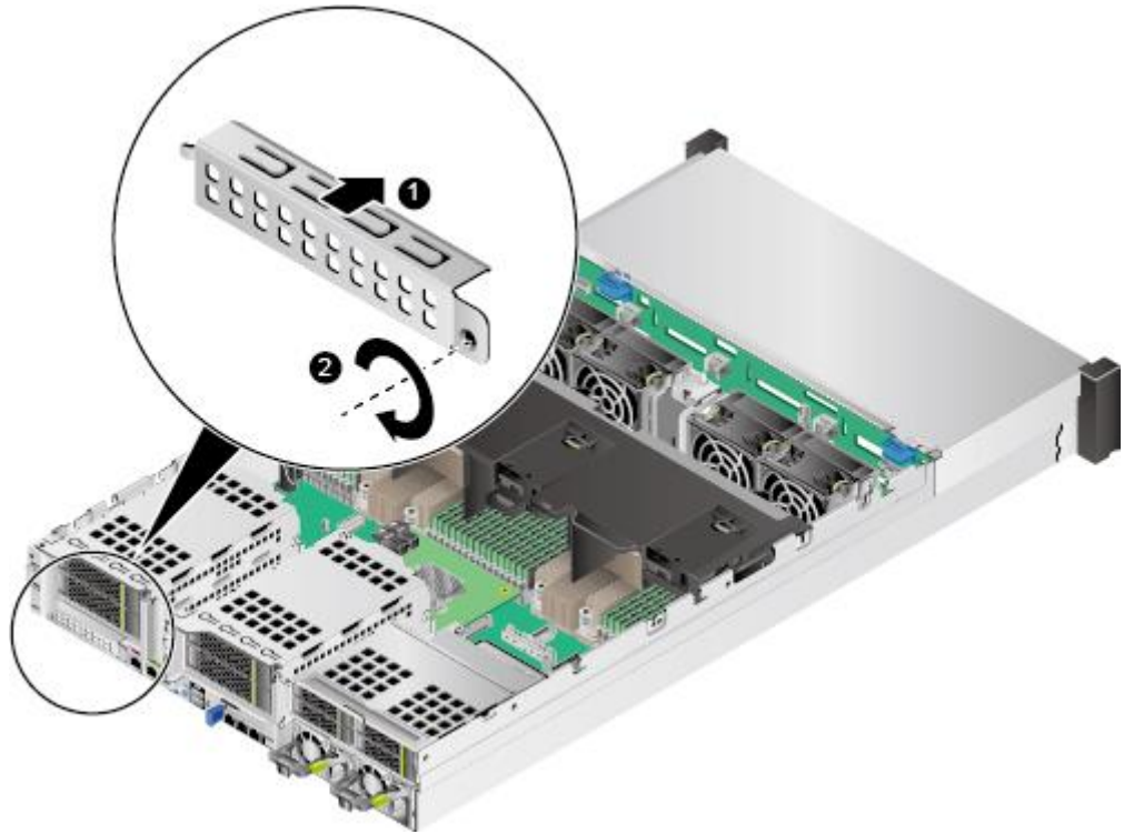
图6-75 安装灵活 IO 卡空闲挡板
