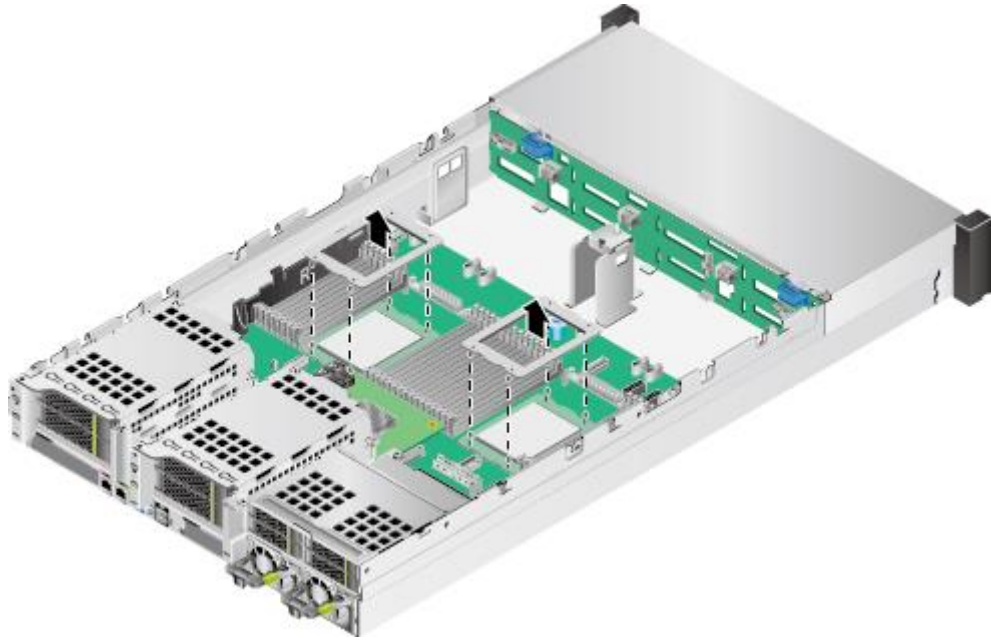
图6-96 拆卸 CPU 托架
