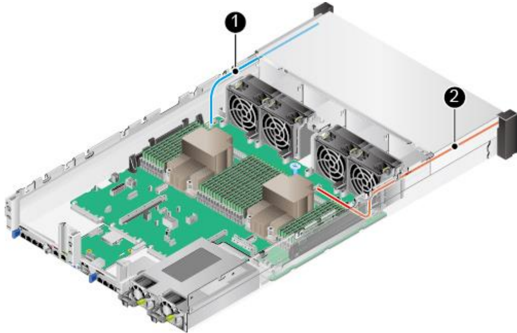
图4-17 左右挂耳连线
