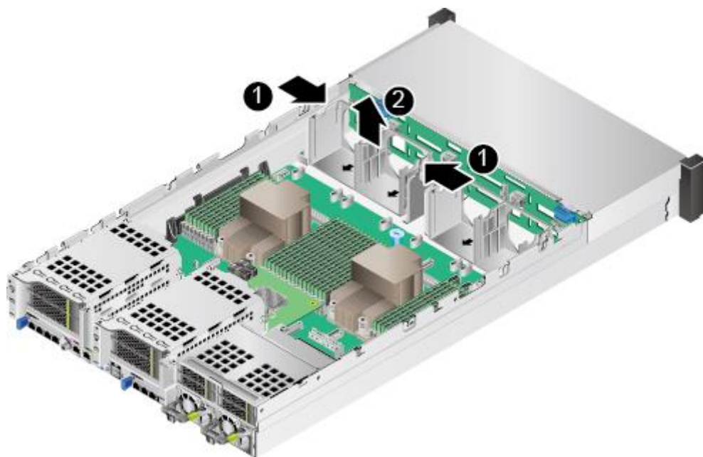
图6-78 拆卸风扇支架
