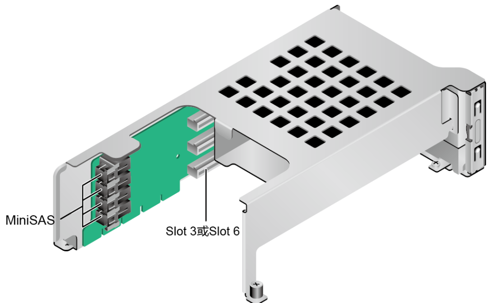
图3-33 Riser 卡 5 (SAS Riser)
