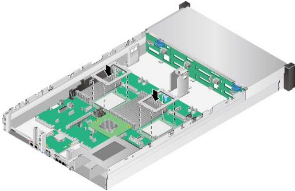
图6-105 安装 CPU 托架
