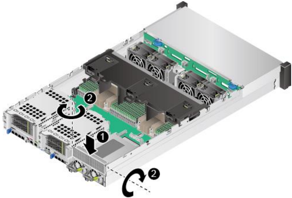
图6-47 安装空闲挡板 (3)
