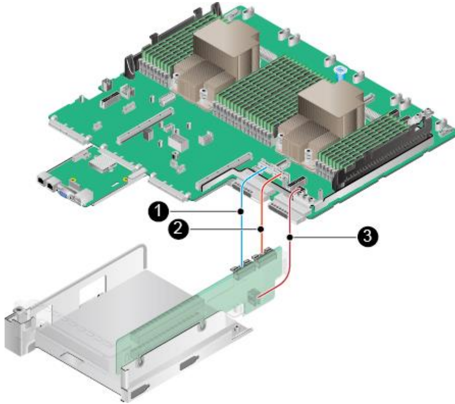
图4-21 IO 模组 3 Riser 卡连线
