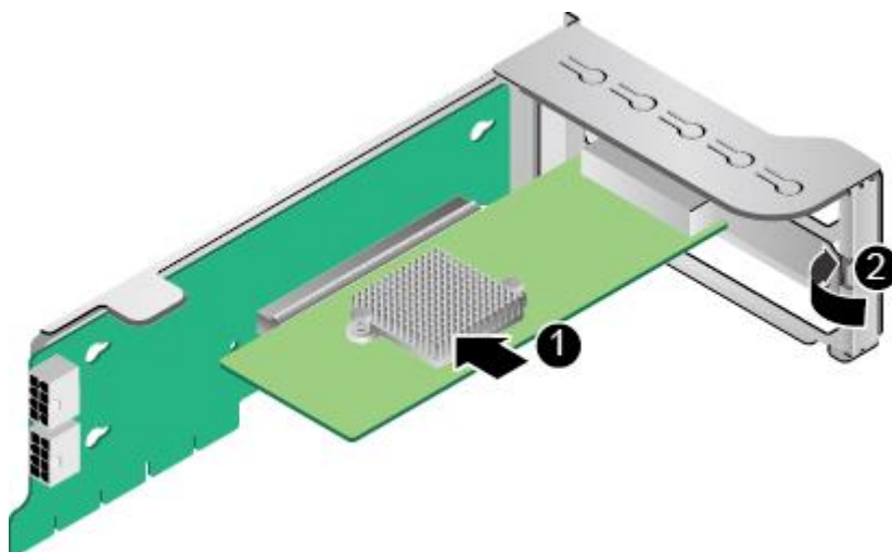
图6-58 安装 Riser 卡上的 PCIe 卡
