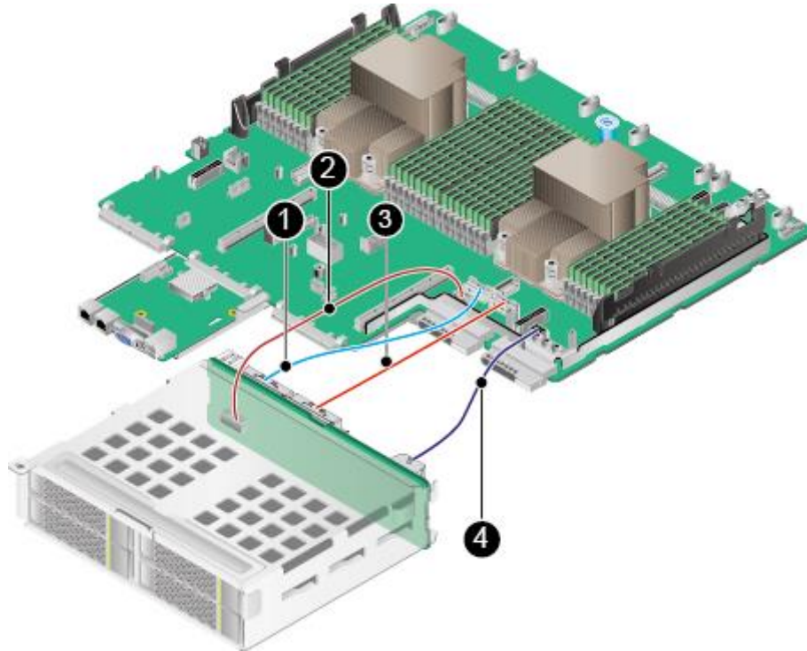
图4-20 IO 模组 3 硬盘背板连线
