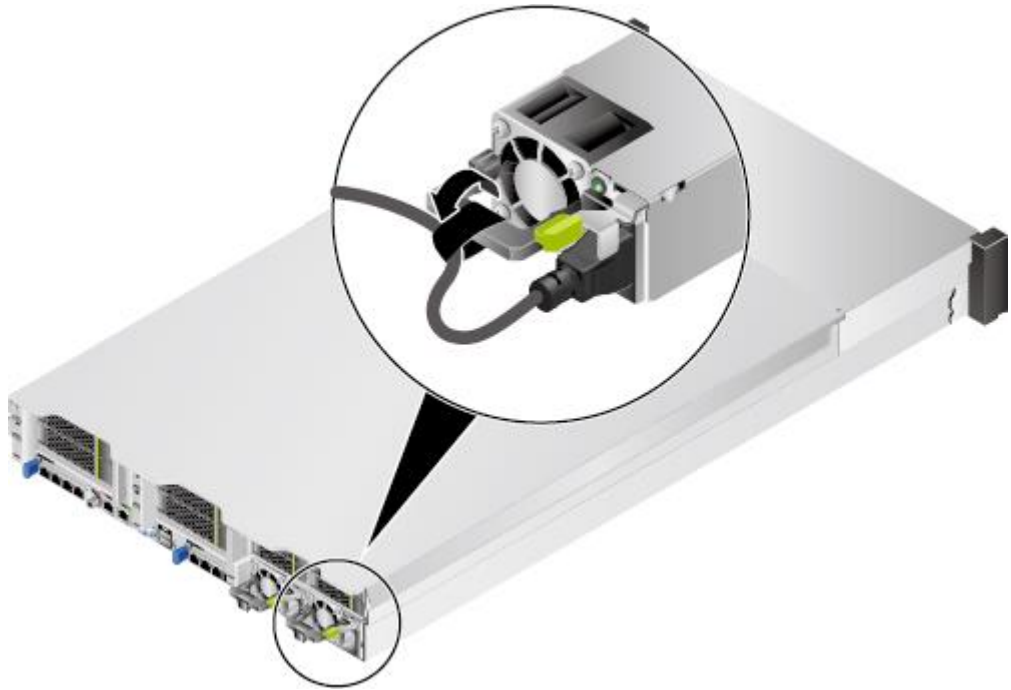
图6-26 固定电源线缆
