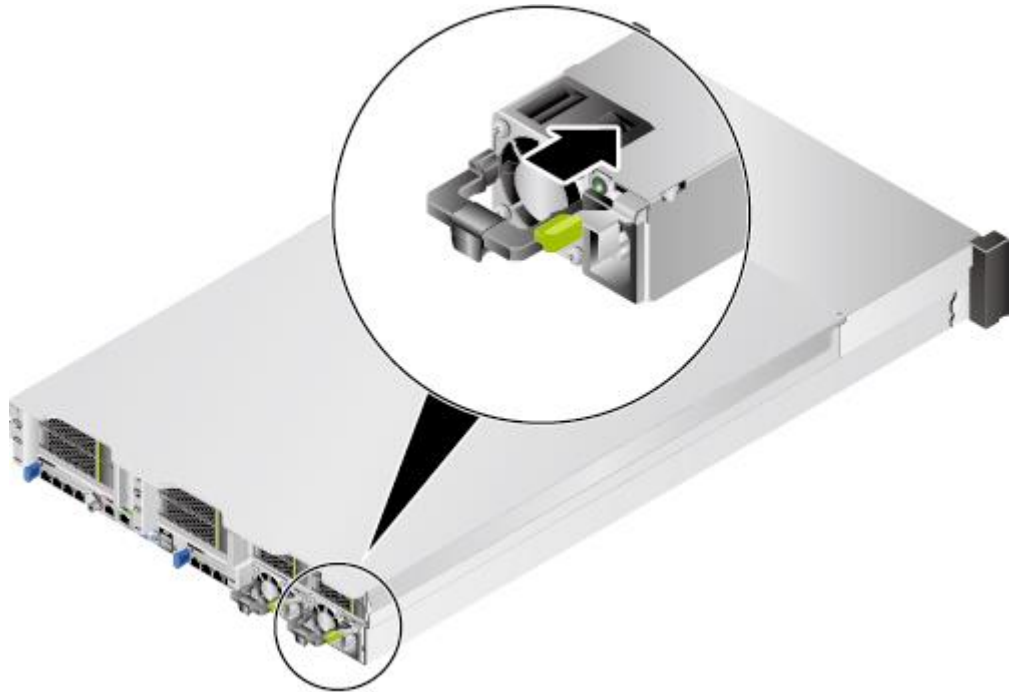
图6-24 安装电源模块
