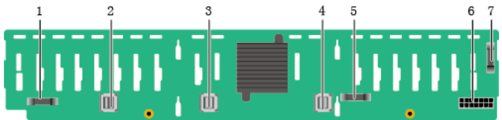
图3-21 25x2.5 英寸硬盘背板
