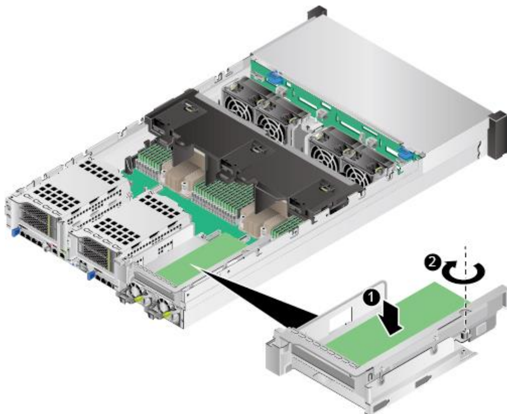
图6-54 安装 Riser 模组 3 的上托架
