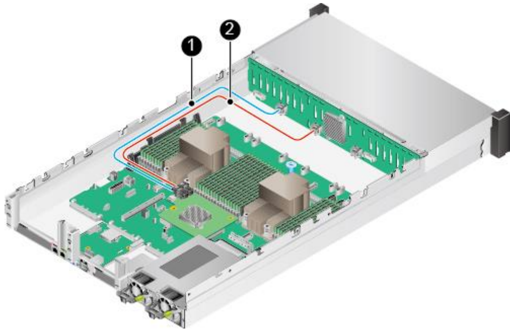
图4-11 前置硬盘背板的 SAS 信号线
