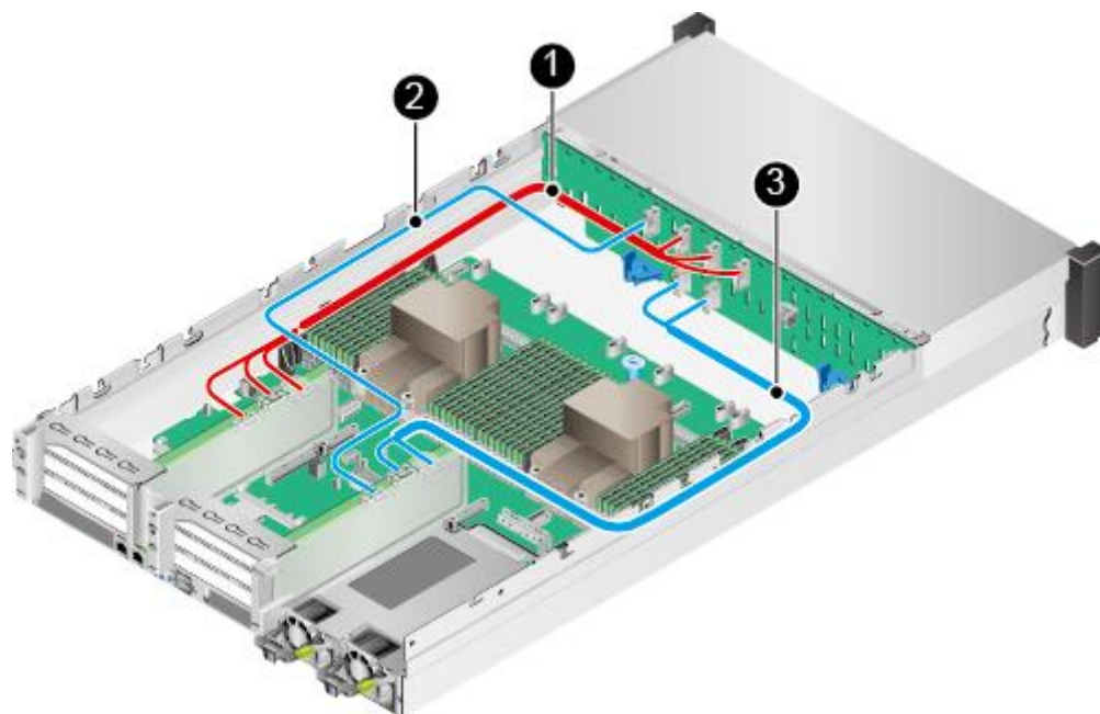
图4-16 NVMe 硬盘扩展适配卡信号线
