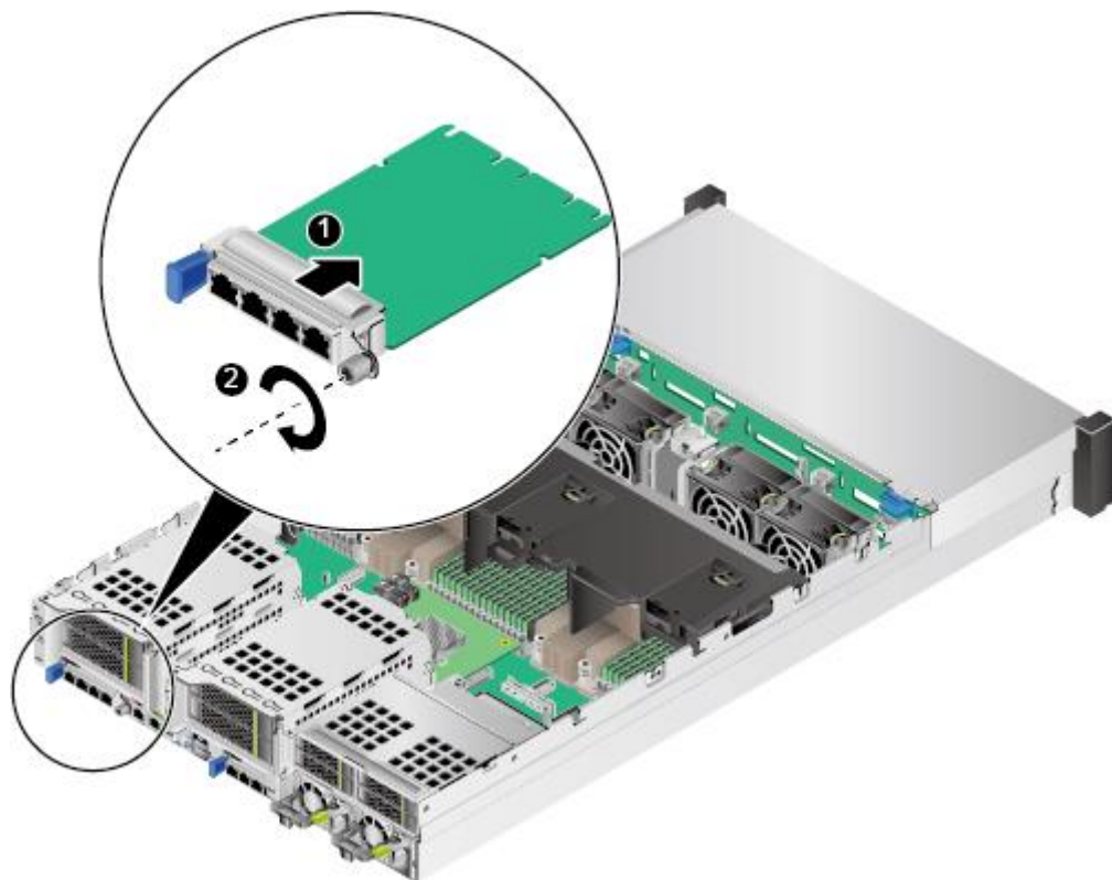
图6-77 安装灵活 IO 卡
