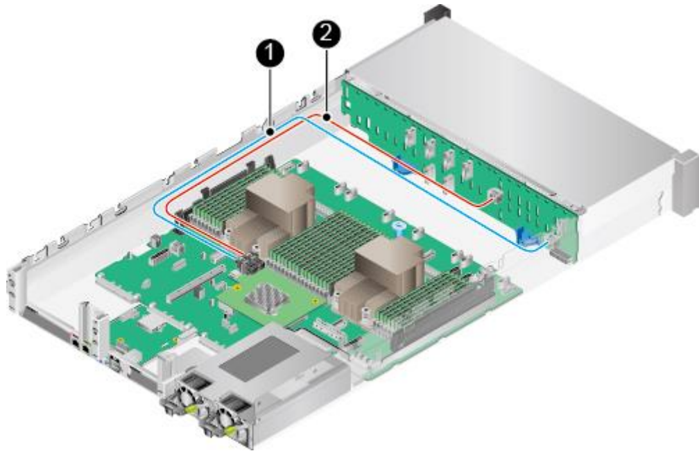
图4-15 前置硬盘背板的 SAS 信号线
