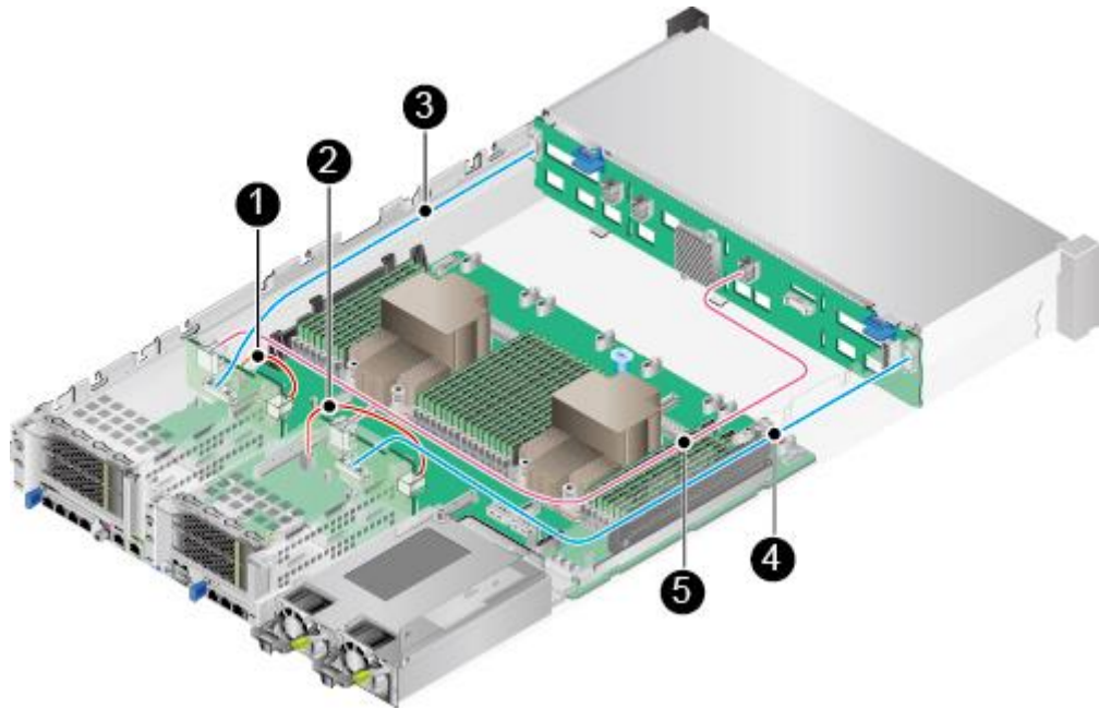
图4-4 后置硬盘背板连线
