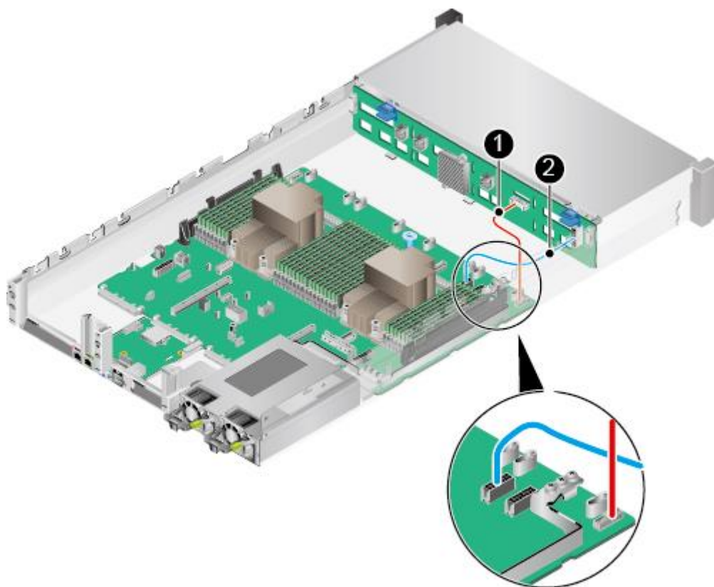
图4-2 前置硬盘背板的电源线和点灯信号线
