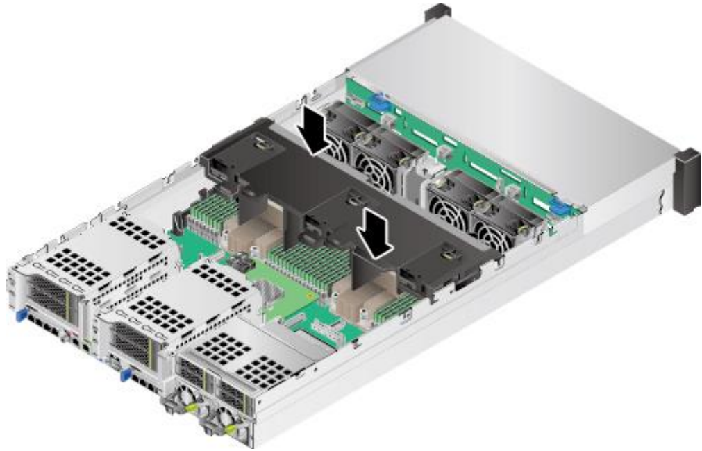
图6-37 安装导风罩
