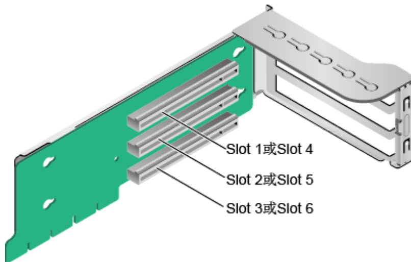
图3-29 Riser 卡 1 (3x8)
