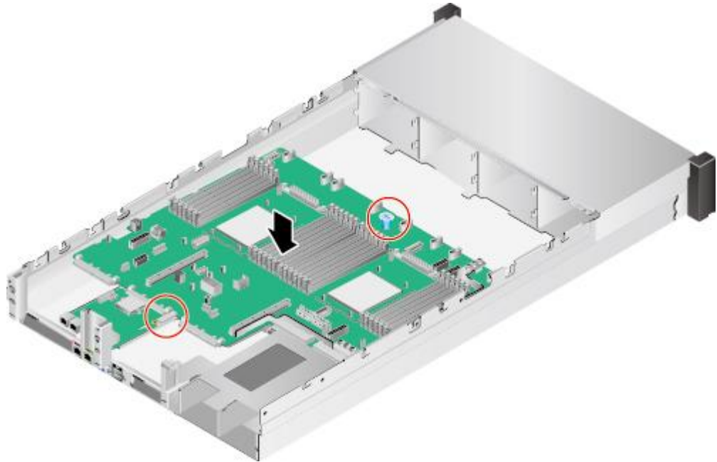
图6-100 安装主板
