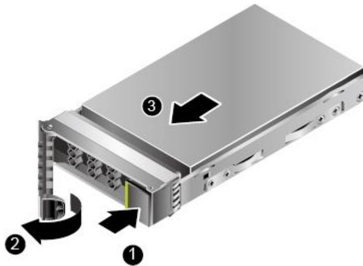
图6-17 拆卸硬盘
