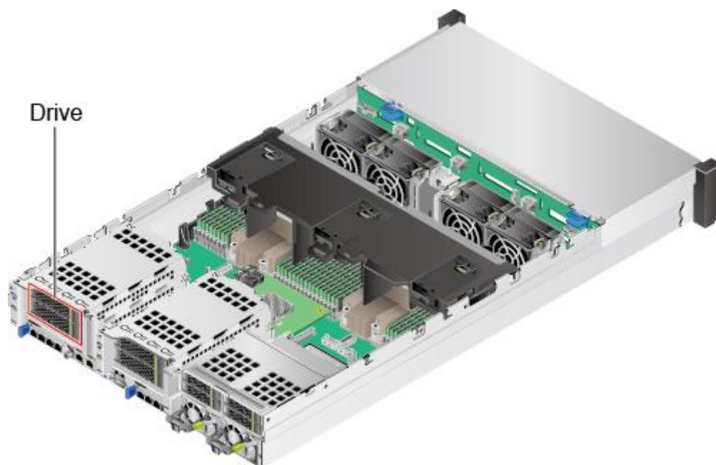
图6-85 硬盘位置
