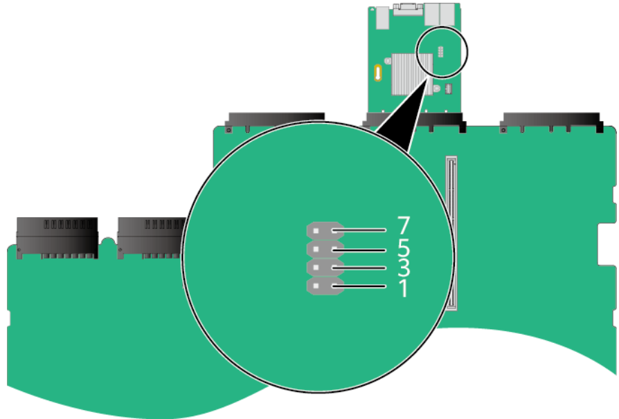
图8-7 跳线位置
