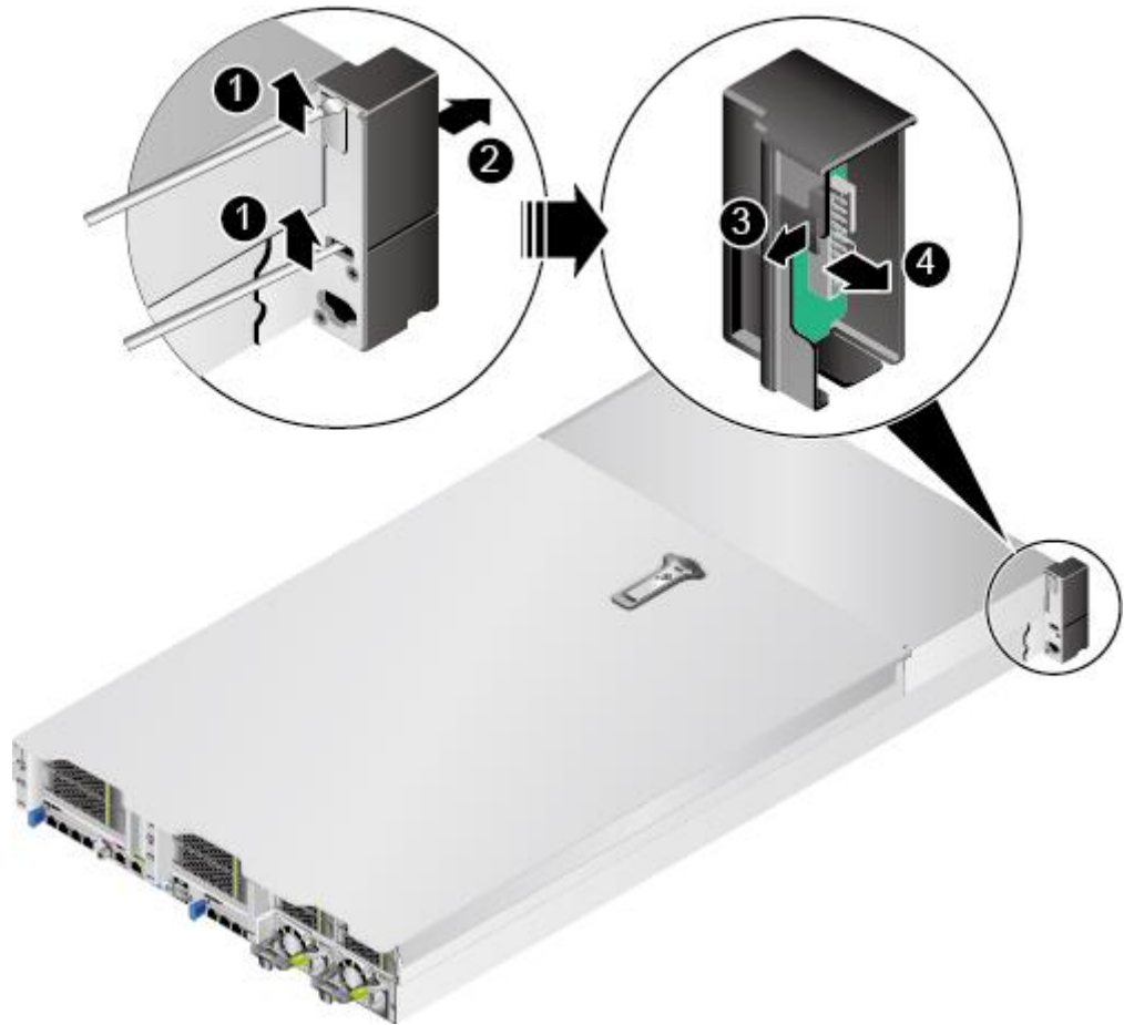
图6-90 拆卸左挂耳板
