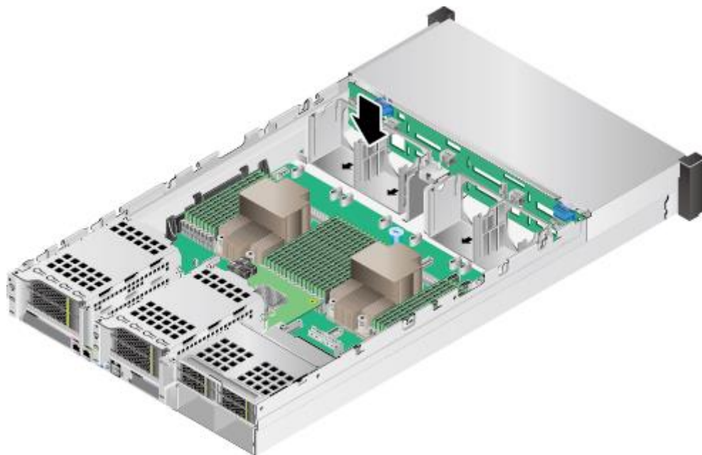
图6-107 安装风扇支架
