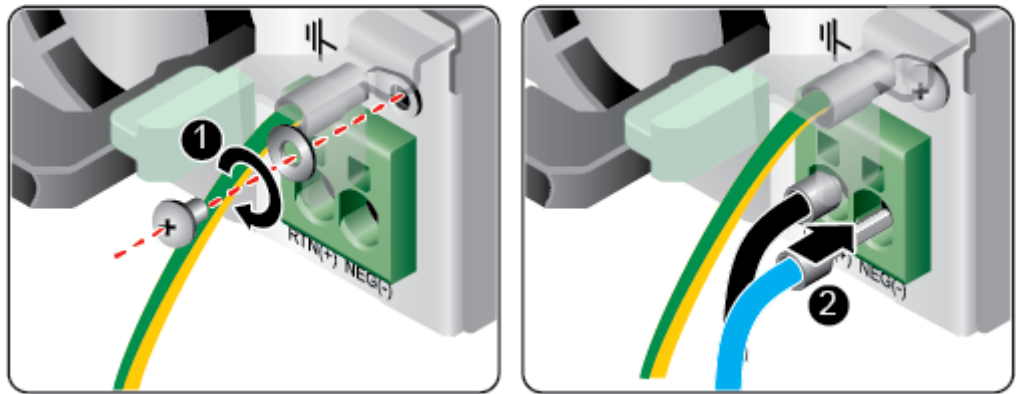
图6-32 连接电源线缆
