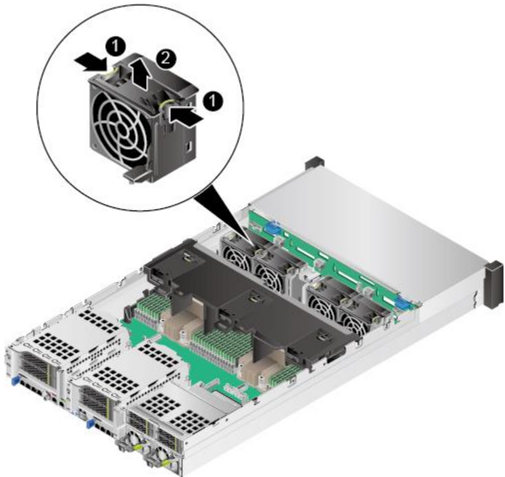
图6-39 拆卸风扇模块
