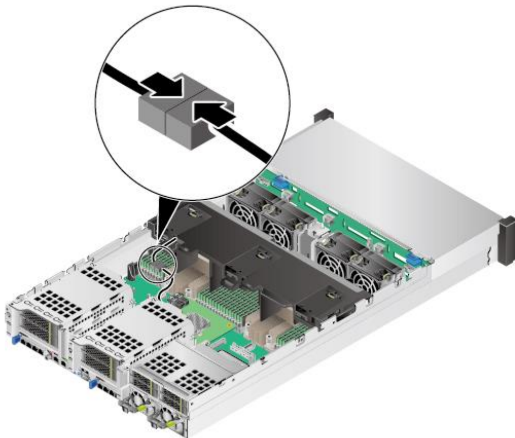
图6-38 连接超级电容线缆
