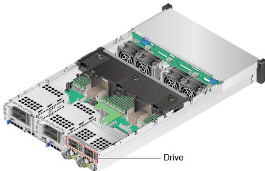
图6-89 硬盘位置
