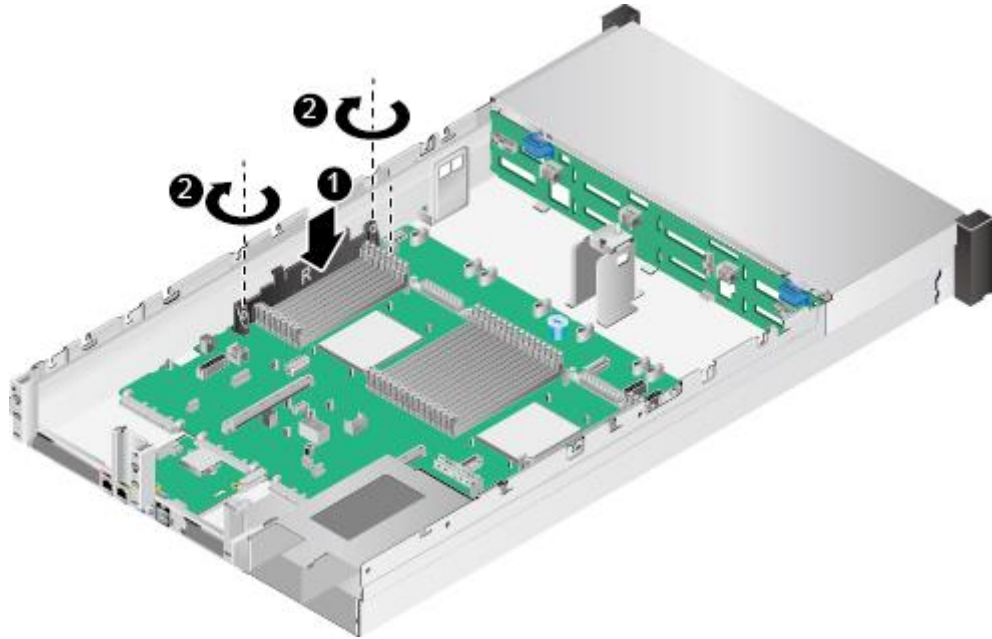
图6-102 安装理线架
