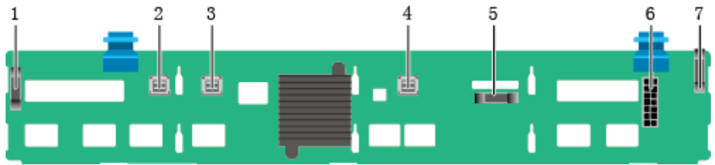
图3-20 12x3.5 英寸 EXP 硬盘背板
