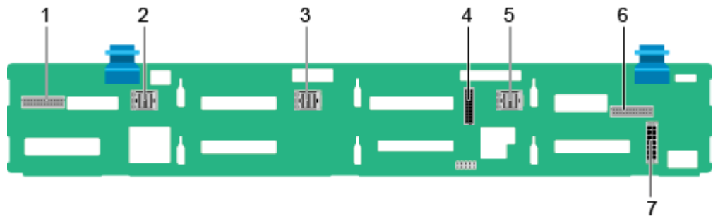
图3-19 12x3.5 英寸直通硬盘背板
