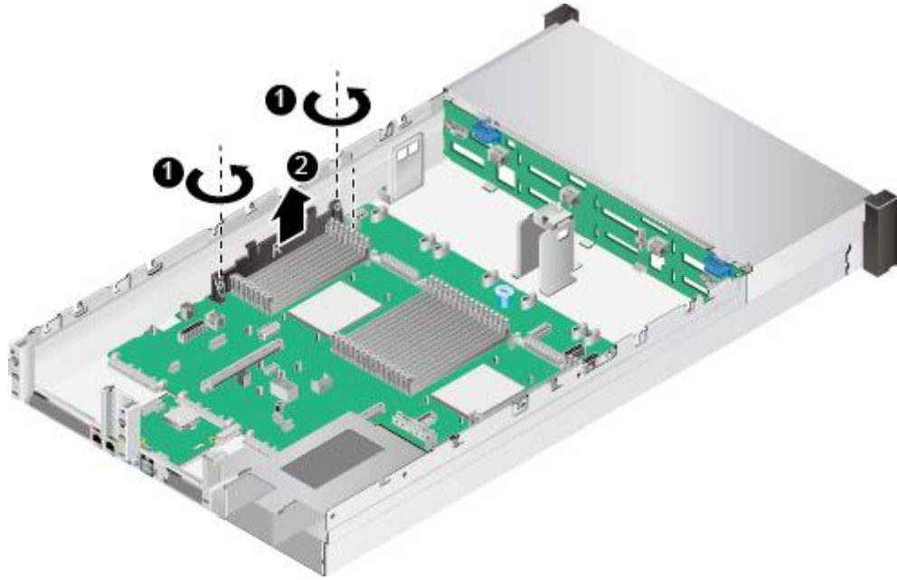
图6-97 拆卸理线架
