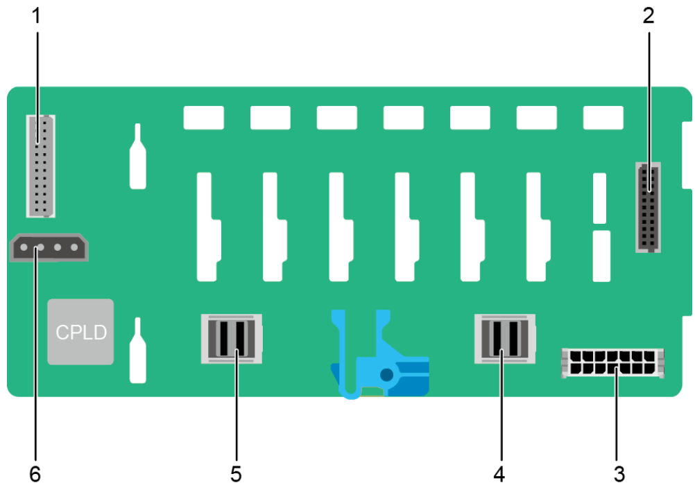
图3-23 8x2.5 英寸硬盘背板
