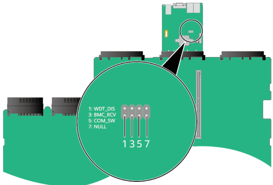
图8-6 跳线位置
