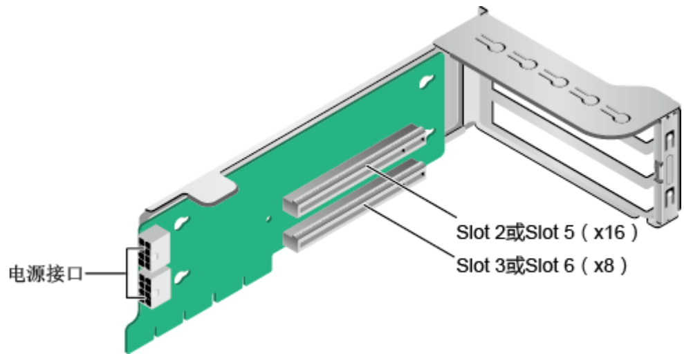
图3-30 Riser 卡 2 (1x8+1x16)
