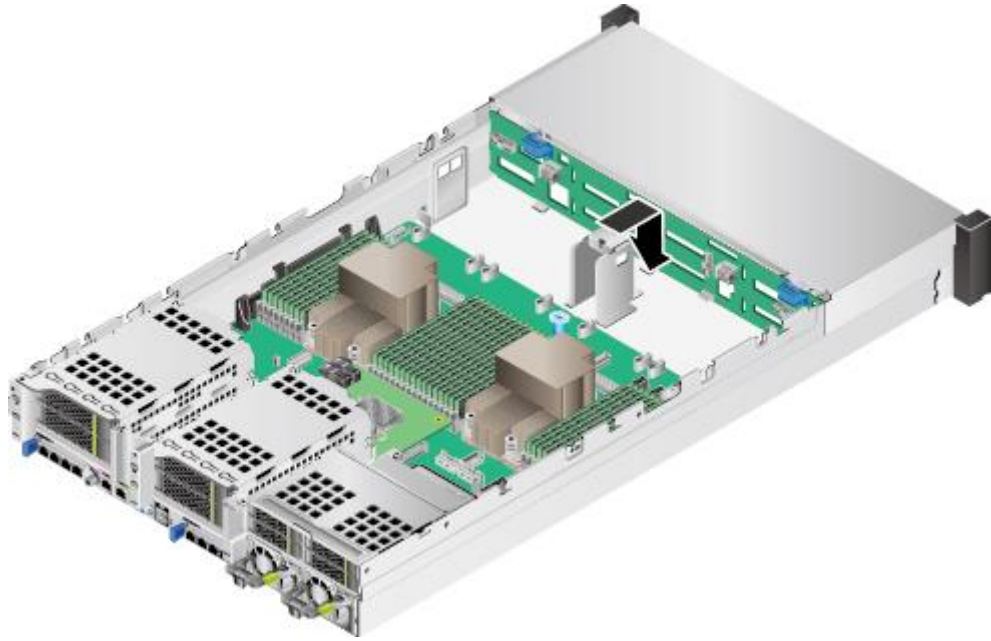
图6-80 安装硬盘背板
