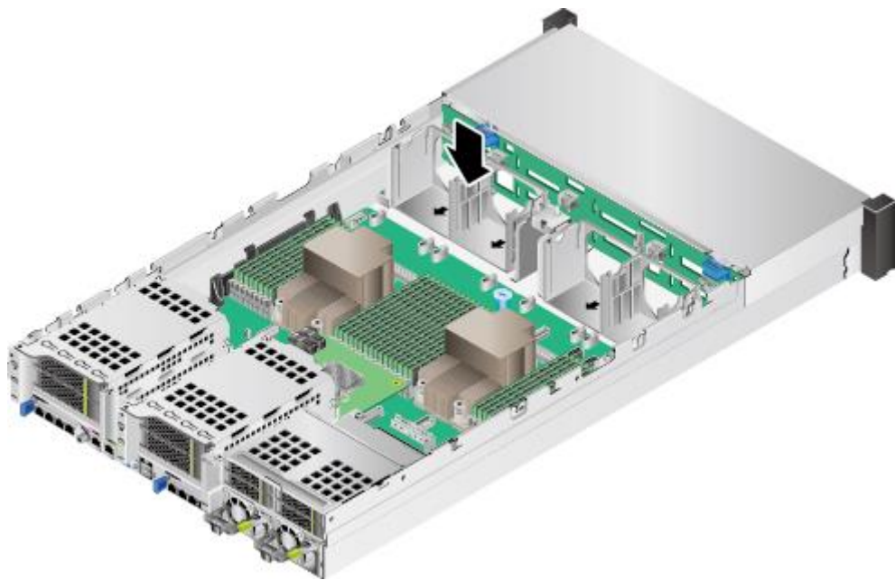
图6-81 安装风扇支架
