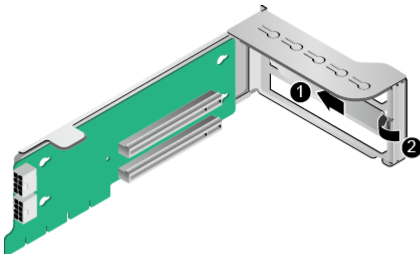
图6-56 安装空闲挡板
