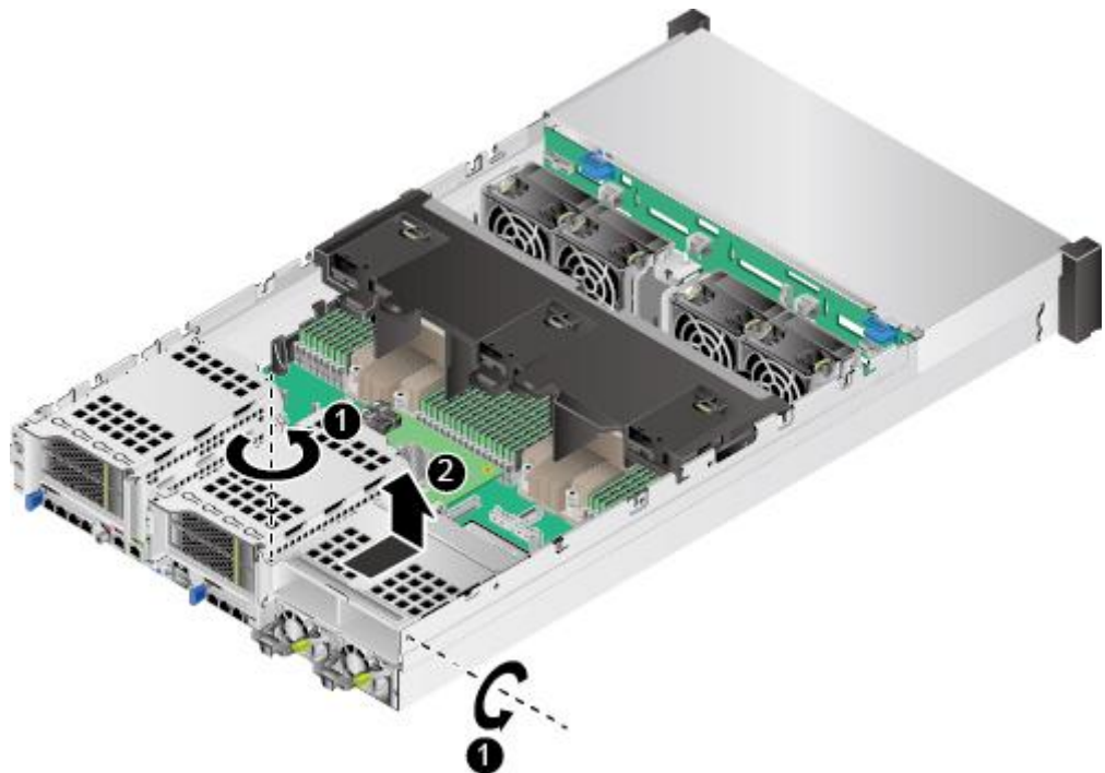
图6-87 拆卸后置硬盘组件
