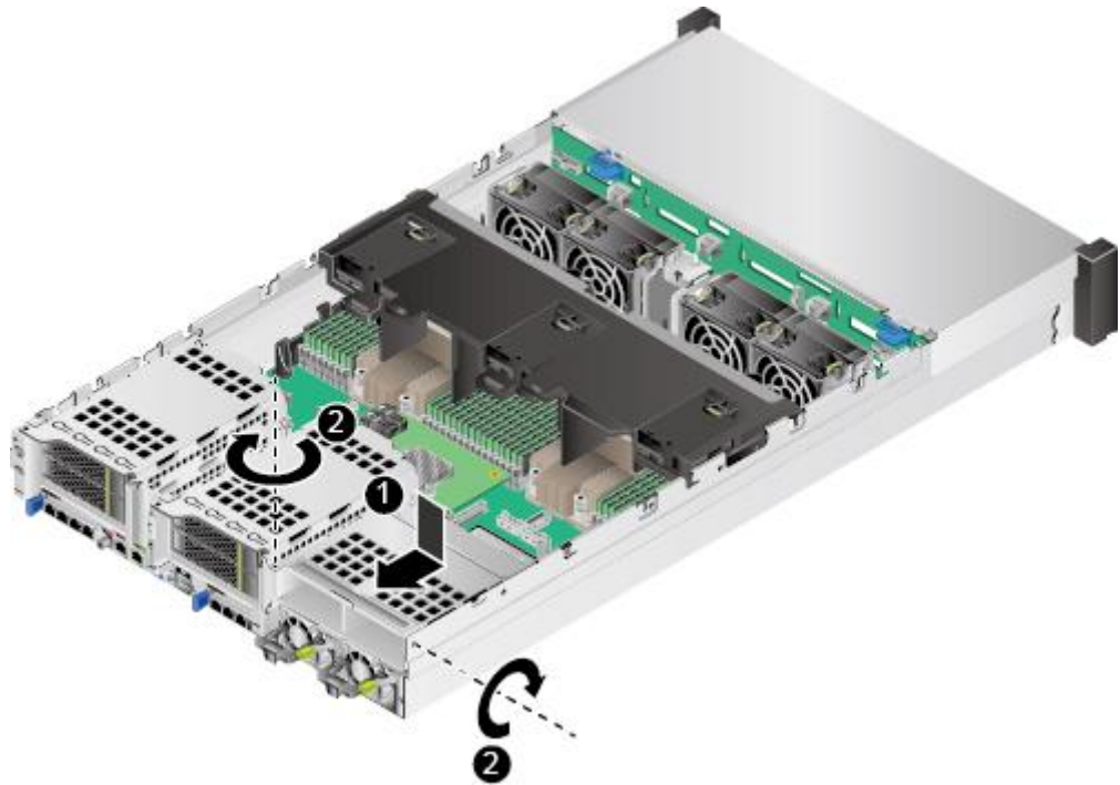
图6-88 安装后置硬盘组件
