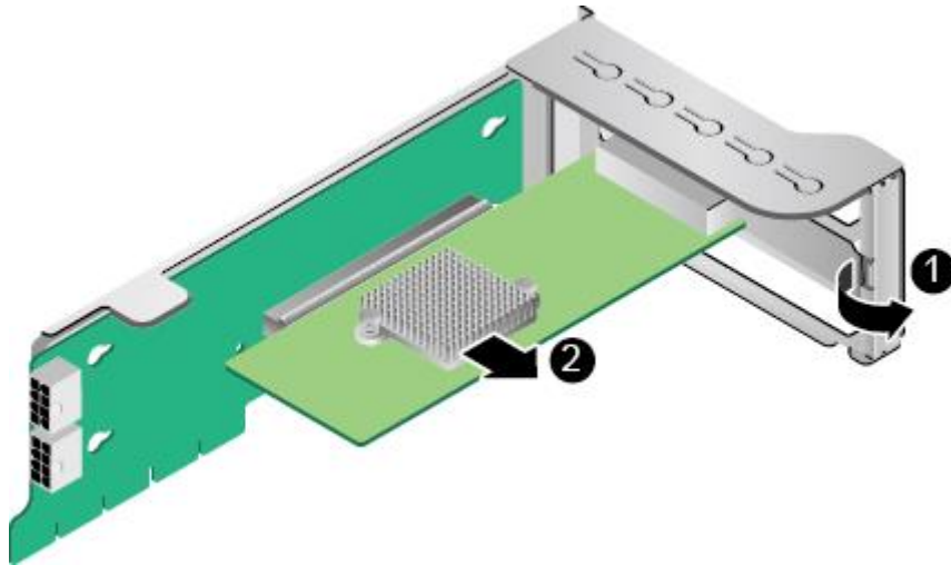
图6-55 拆卸 Riser 卡上的 PCIe 卡
