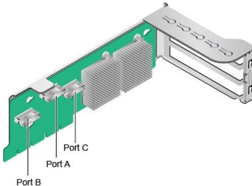
图3-31 Riser 卡 3 (12NVMe 专用)
