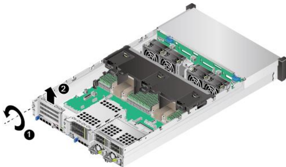
图6-48 拆卸空闲挡板 (1)
