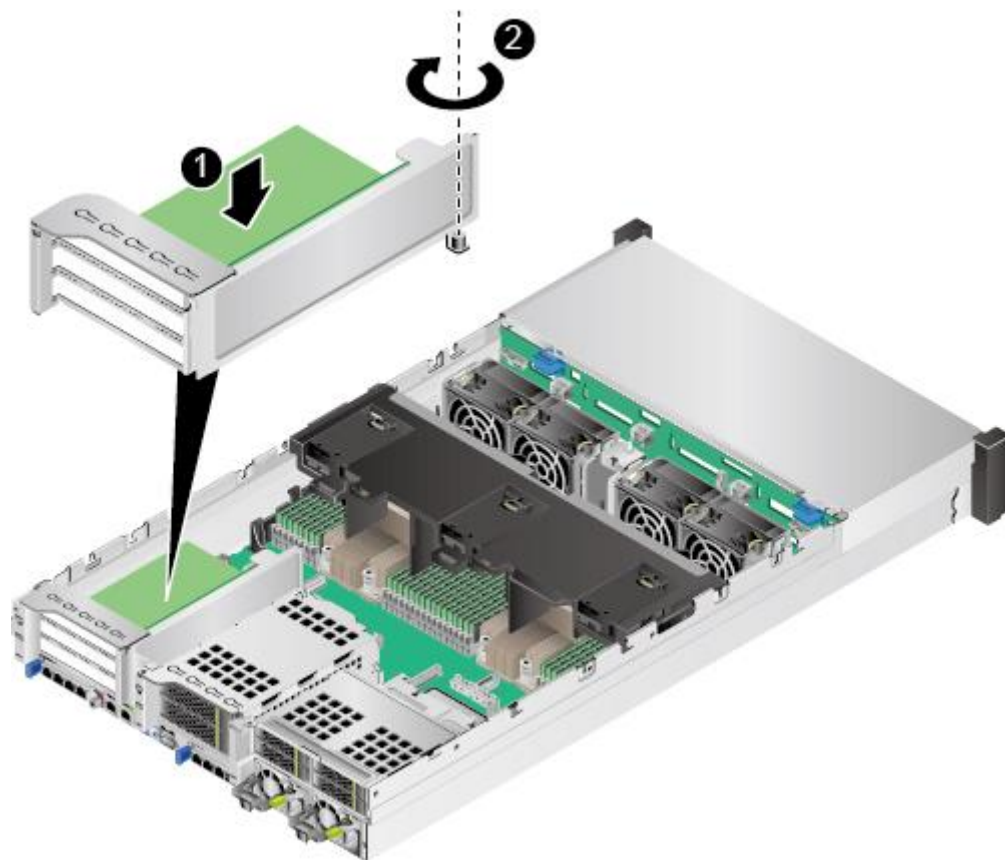
图6-51 安装 Riser 模组 1
