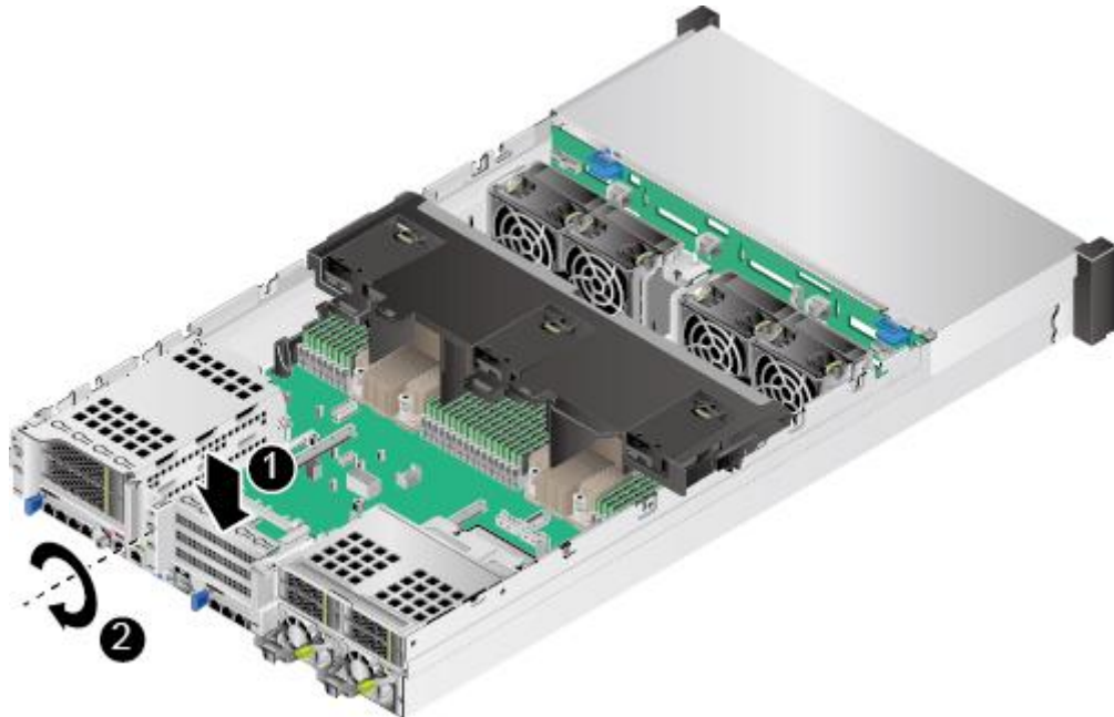
图6-46 安装空闲挡板（2）
