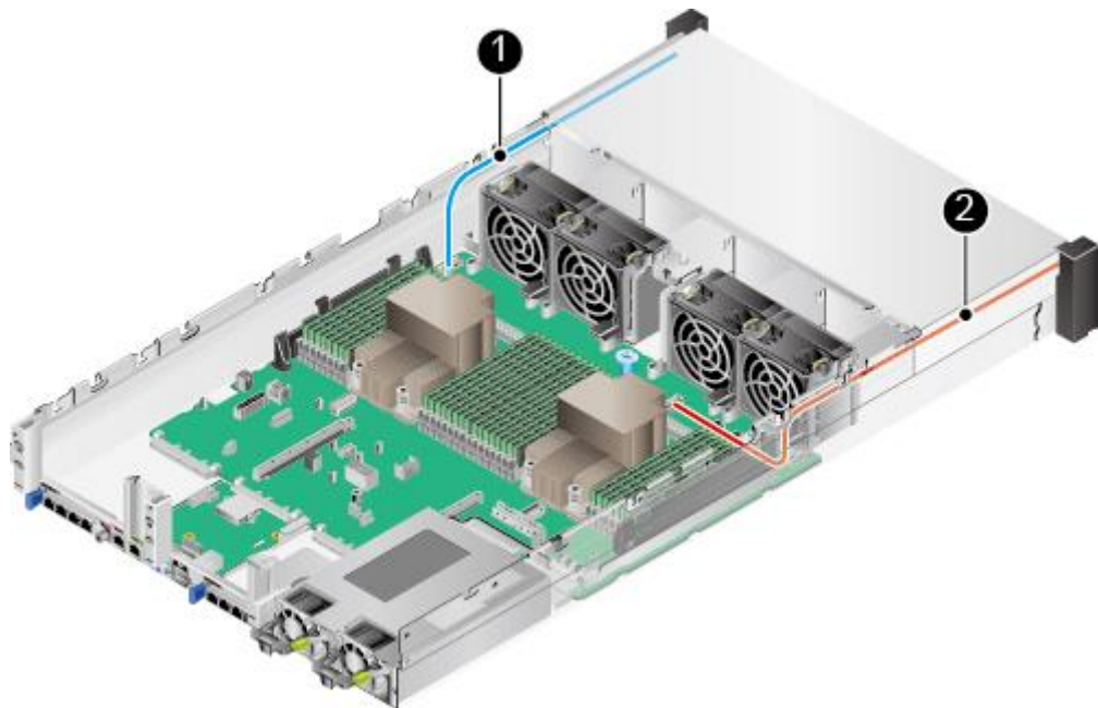
图4-1 左右挂耳连线
