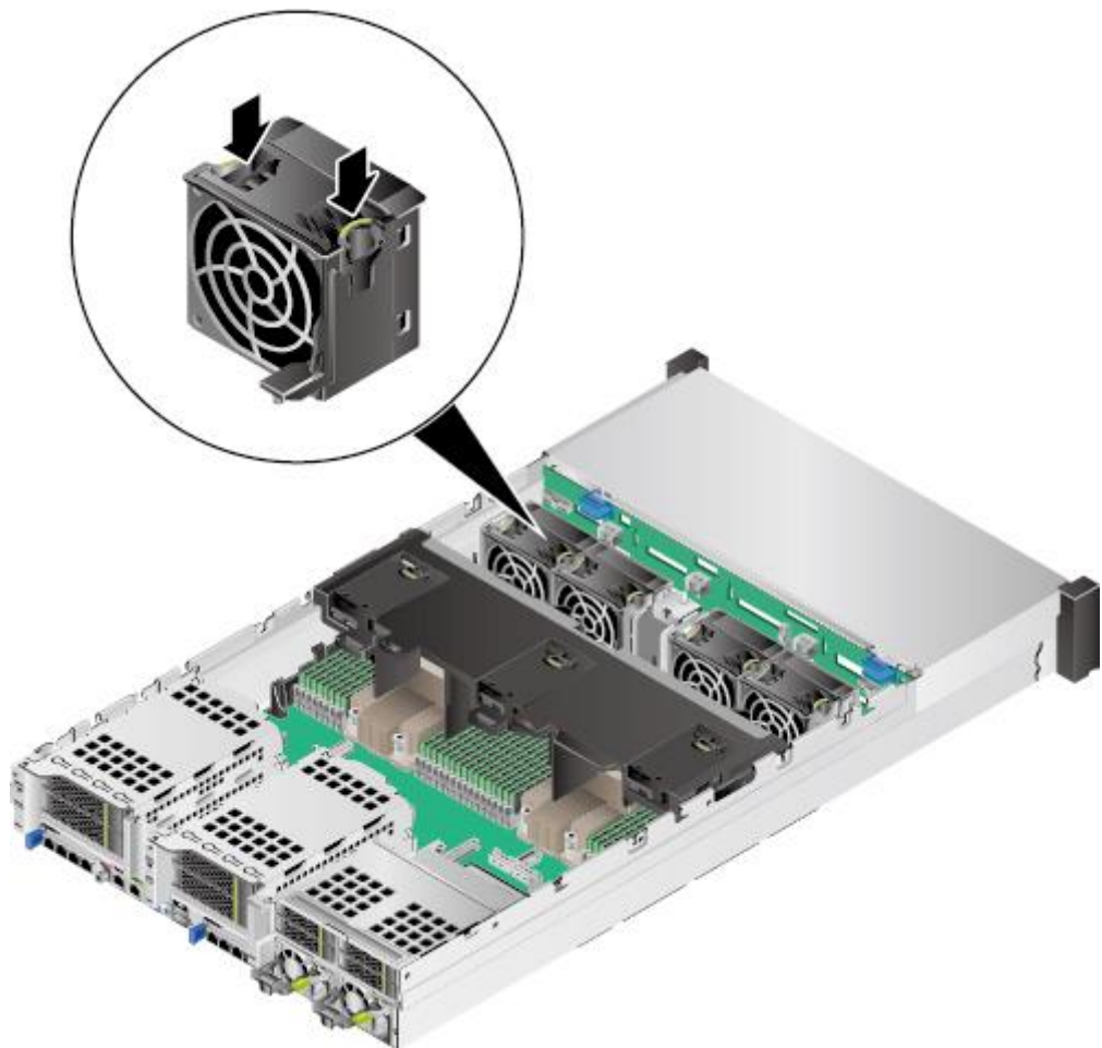
图6-40 安装风扇模块
