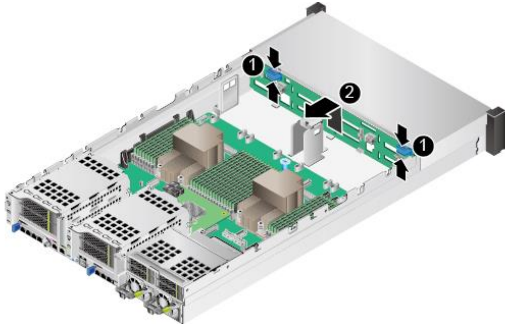
图6-79 拆卸硬盘背板
