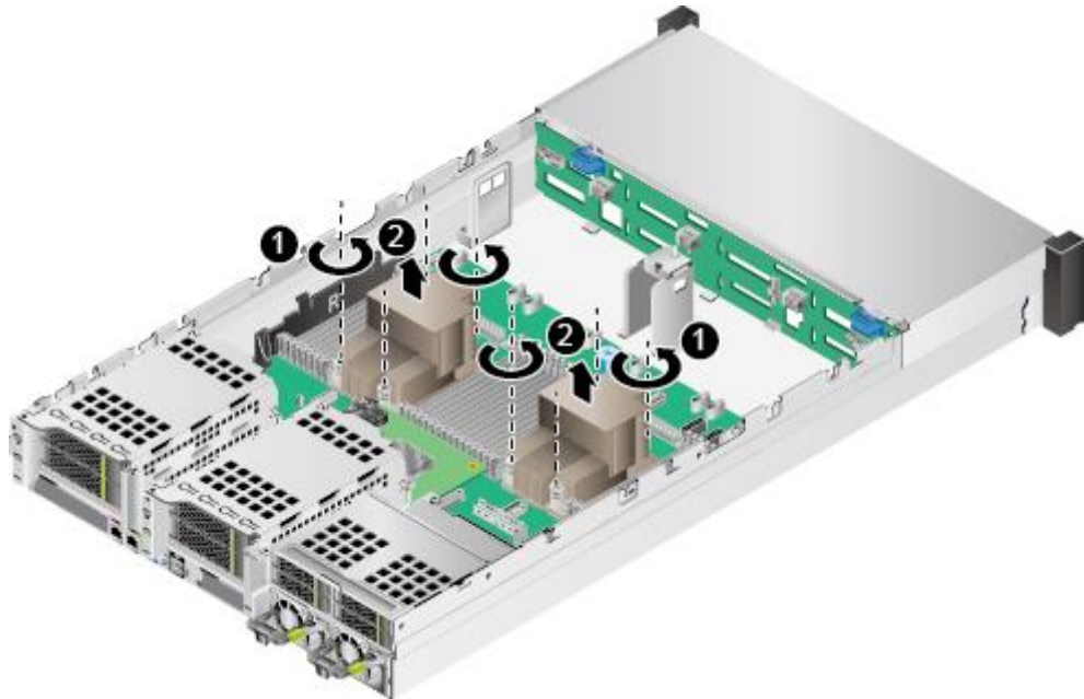
图6-95 拆卸 CPU 散热器
