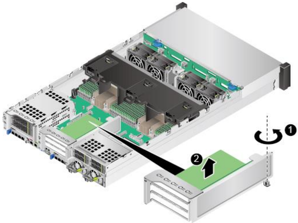
图6-42 拆卸 Riser 模组 2
