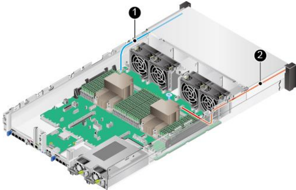
图4-5 左右挂耳连线
