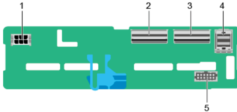
图3-26 4x2.5 英寸后置硬盘背板
