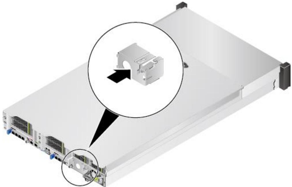
图6-22 安装电源空闲挡板
