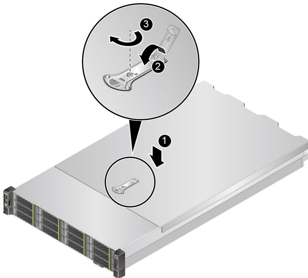
图6-34 安装机箱盖
