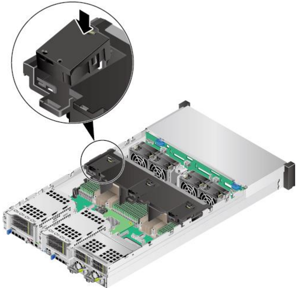
图6-69 安装超级电容支架
