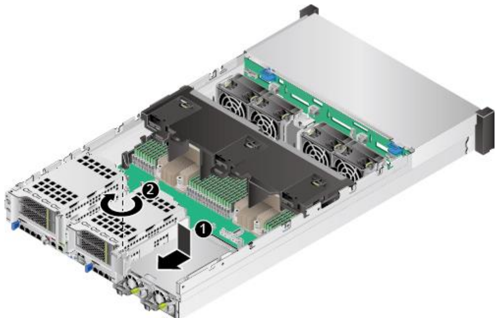
图6-53 安装 Riser 模组 3 的下托架
