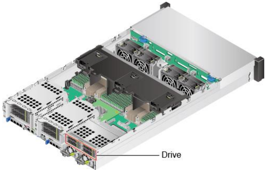
图6-86 硬盘位置
