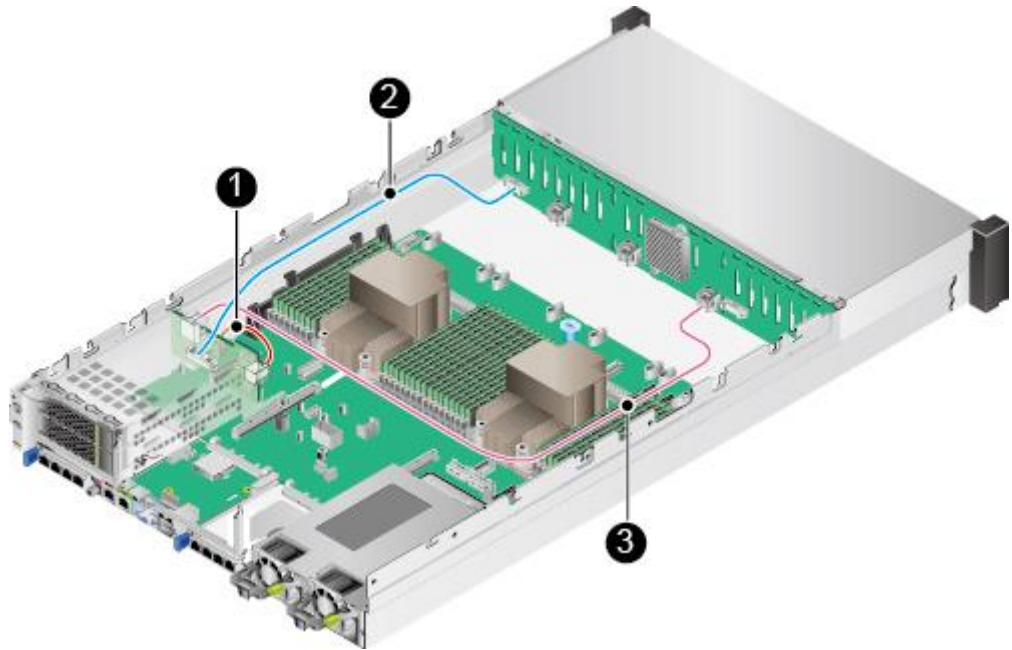
图4-12 后置硬盘背板连线
